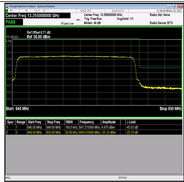
Band5_3MHz_16QAM_20635_15RB#0
