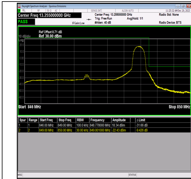
Band5_3MHz_16QAM_20635_1RB#14
