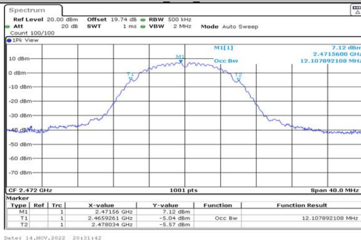
11B_Ant1_2472
