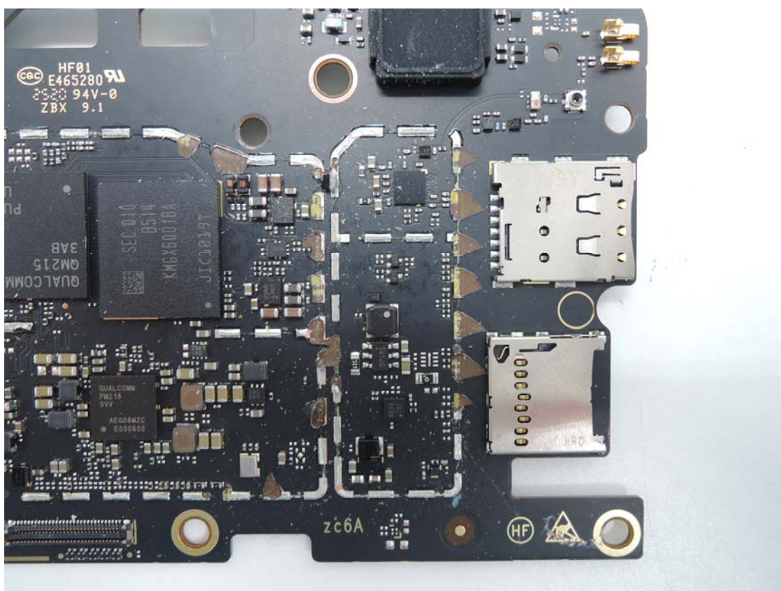
IC Details 3
