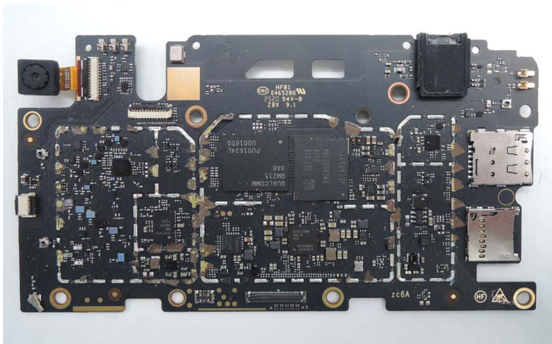
IC Details 2
