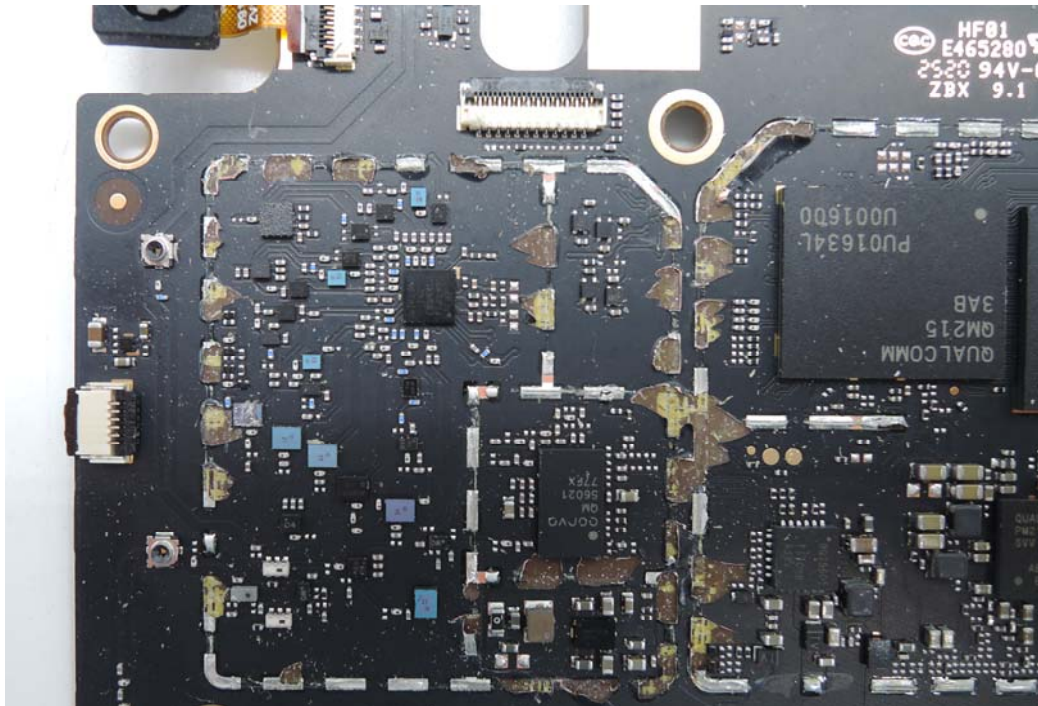
IC Details 4
