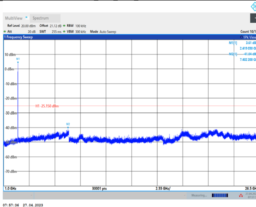
11G_Ant1_2417_0~Reference
