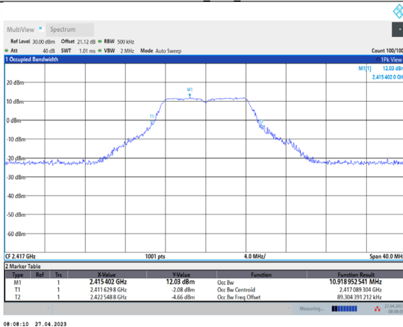
11N20SISO_Ant2_2417
