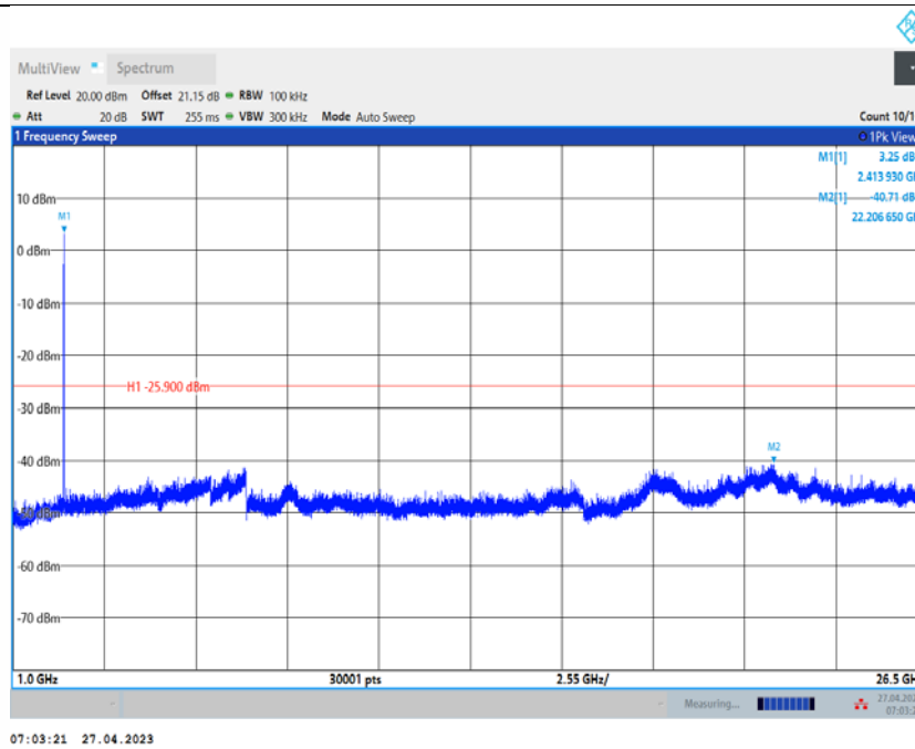
11B_Ant2_2417_0~Reference
