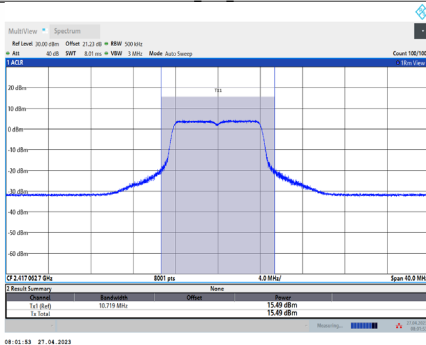
11N20SISO_Ant1_2417
