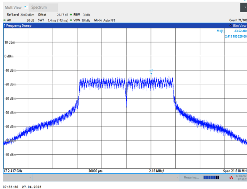
11G_Ant1_2417
