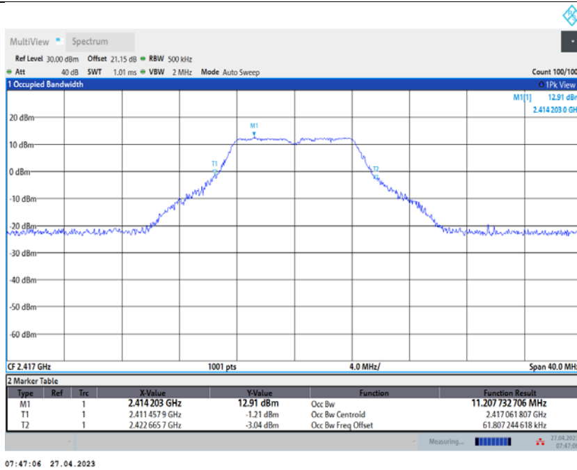
11N20SISO_Ant2_2417
