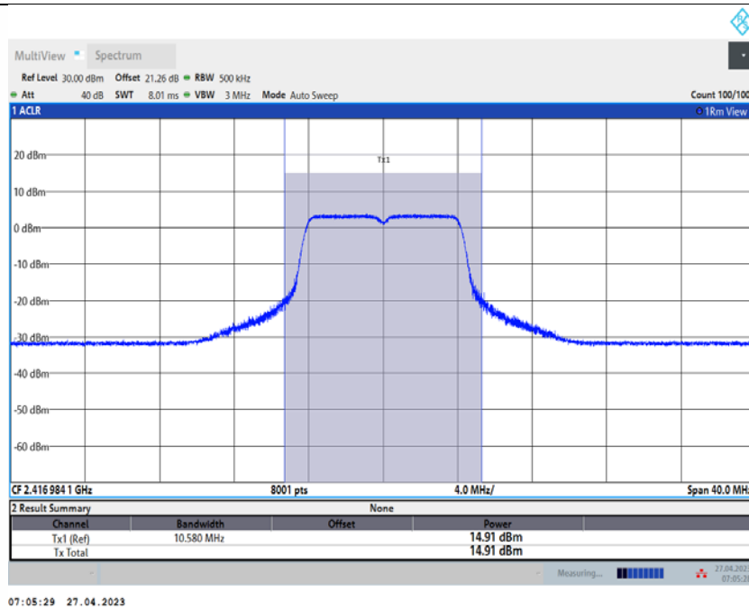
11G_Ant2_2417
