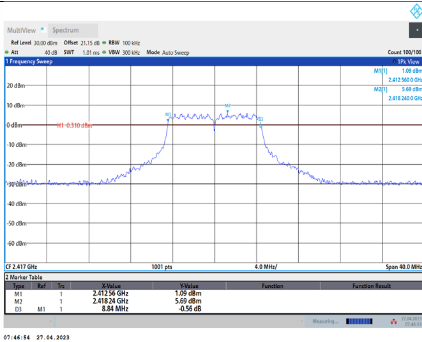
11N20SISO_Ant2_2417
