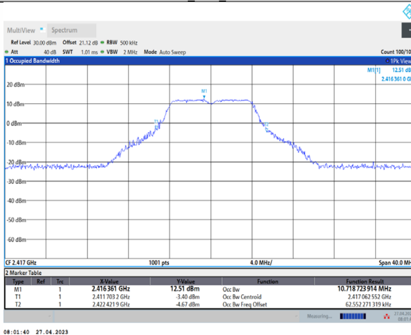
11N20SISO_Ant1_2417
