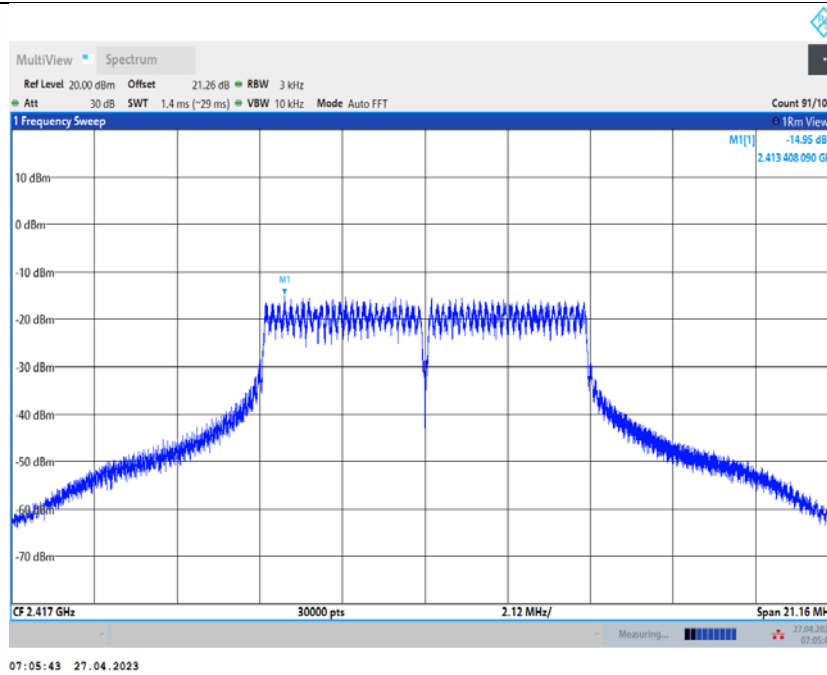
11G_Ant2_2417
