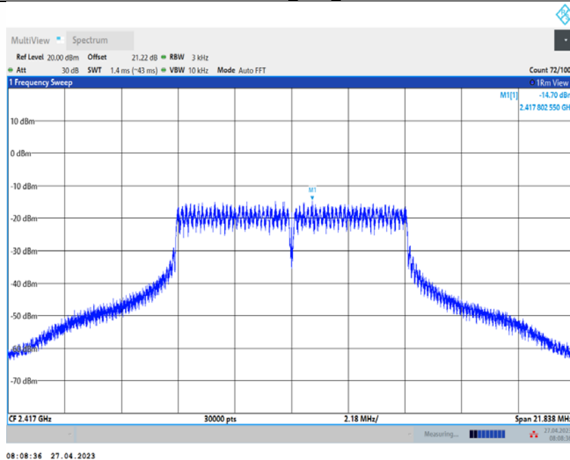
11N20SISO_Ant2_2417
