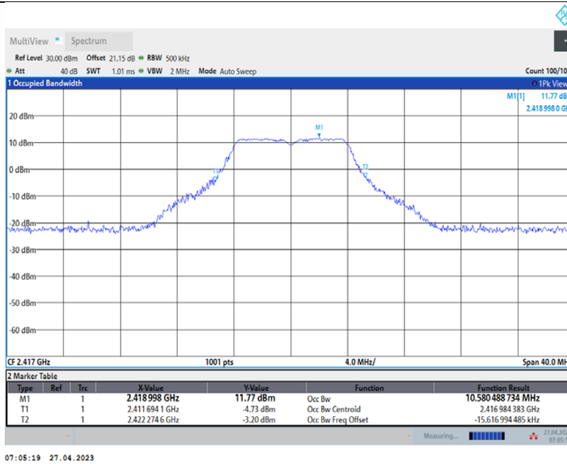
11G_Ant2_2417
