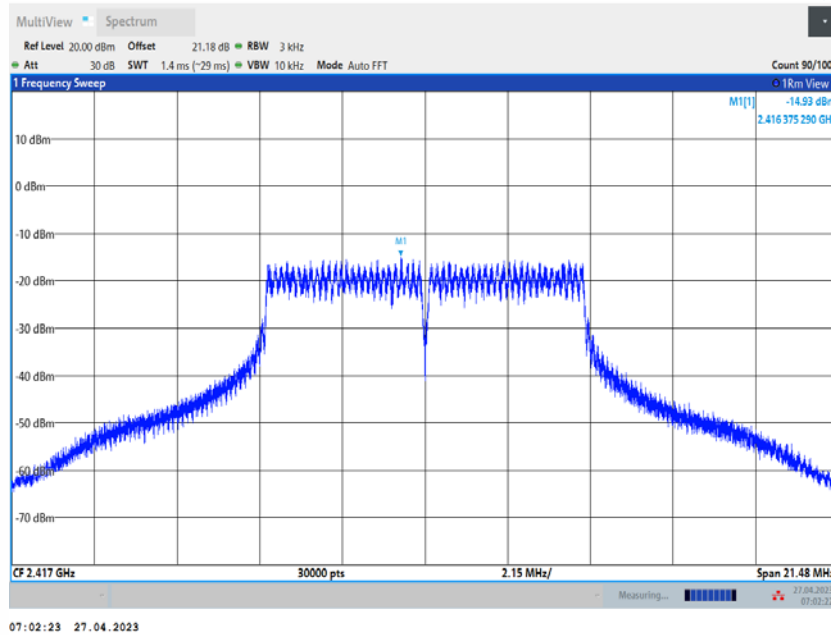
11B_Ant2_2417
