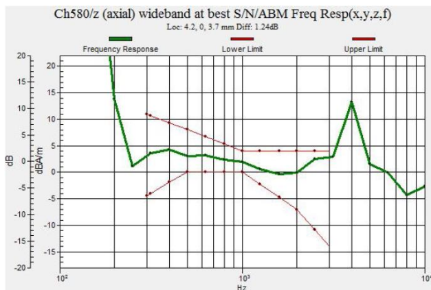
Fig 7.1 CDMA2000 BC10 Ch580
