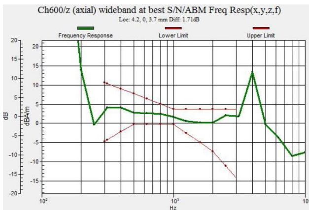
Fig 7.3 CDMA2000 BC1 Ch600
