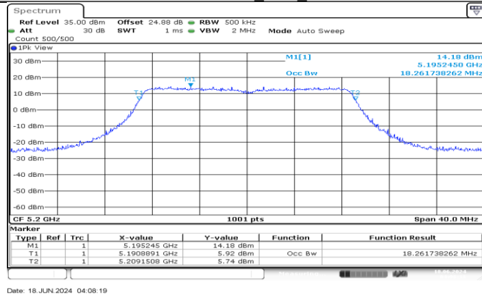
11AC20MIMO_Ant1_5200
