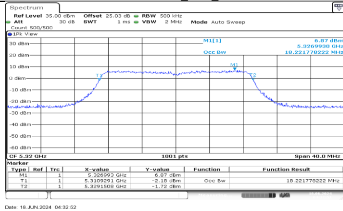
11AC20MIMO_Ant3_5320
