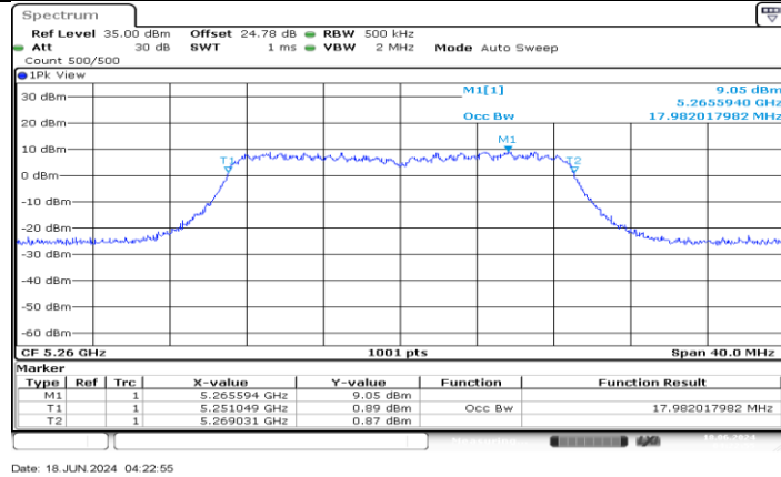
11AC20MIMO_Ant4_5260
