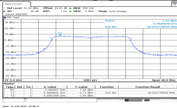
11AC20MIMO_Ant3_5500
