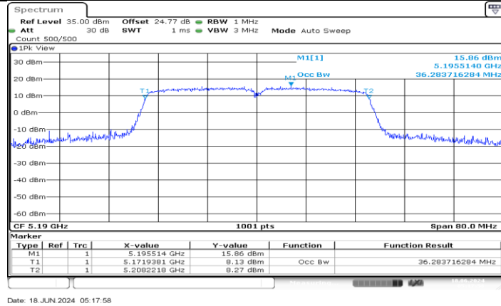
11AC40MIMO_Ant2_5190
