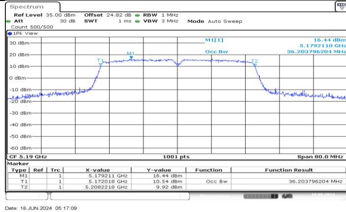
11AC40MIMO_Ant1_5190
