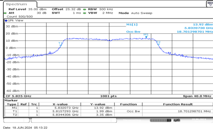
11AC20MIMO_Ant3_5825
