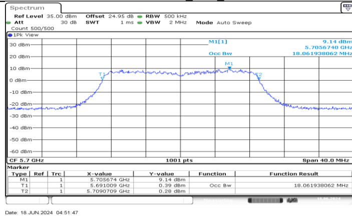
11AC20MIMO_Ant4_5700
