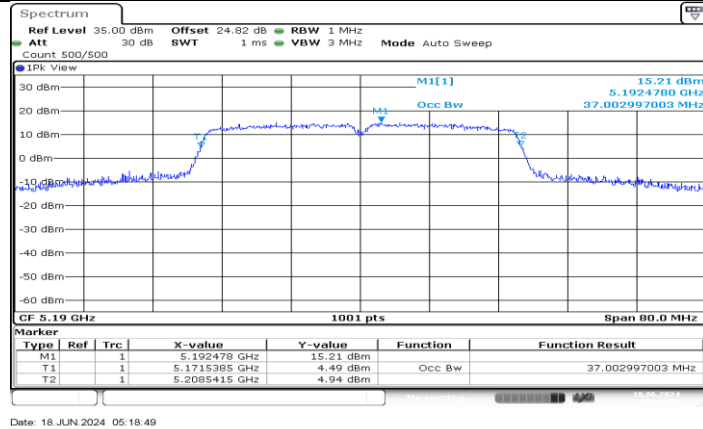
11AC40MIMO_Ant3_5190
