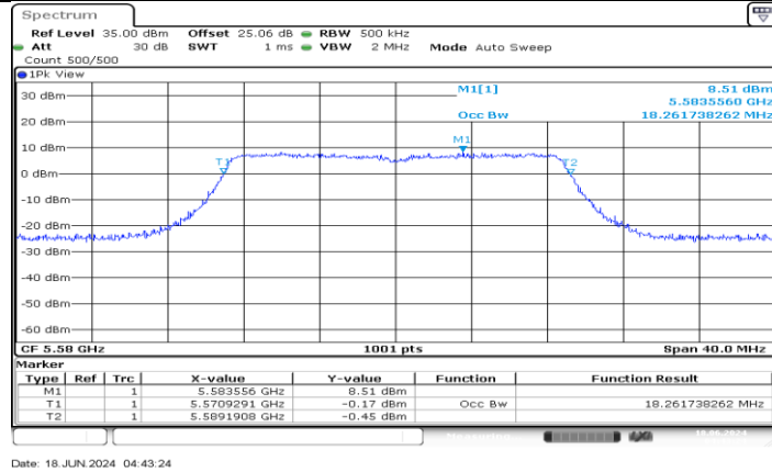
11AC20MIMO_Ant1_5580
