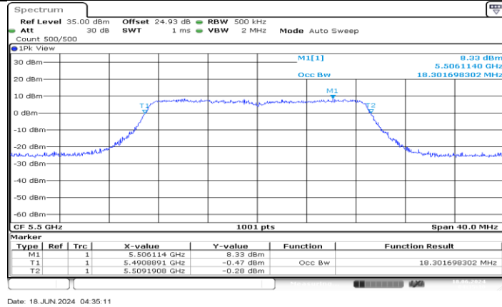
11AC20MIMO_Ant1_5500
