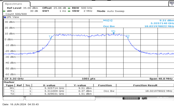
11AC20MIMO_Ant4_5320
