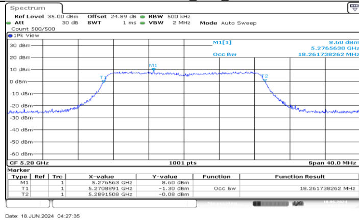
11AC20MIMO_Ant1_5280
