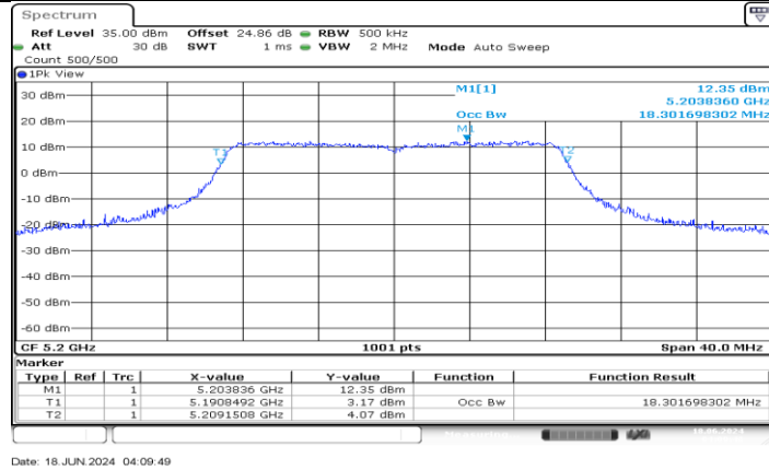
11AC20MIMO_Ant3_5200
