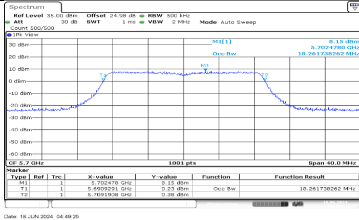
11AC20MIMO_Ant1_5700
