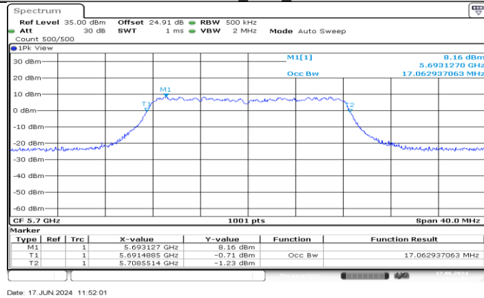
11A-CDD_Ant3_5700
