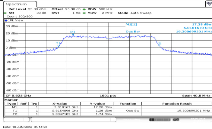
11AC20MIMO_Ant4_5825
