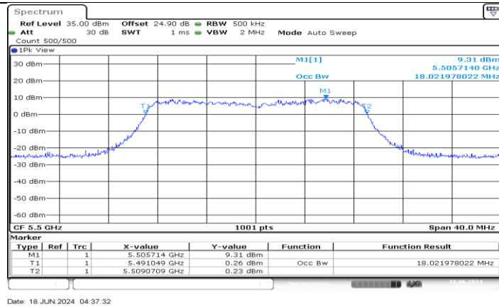
11AC20MIMO_Ant4_5500
