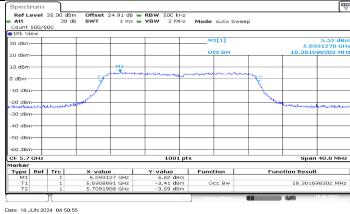
11AC20MIMO_Ant3_5700
