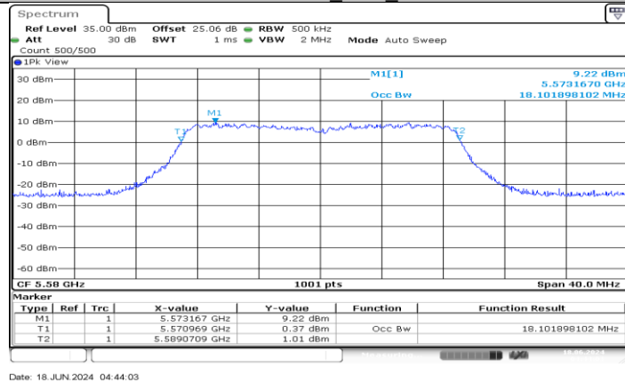
11AC20MIMO_Ant2_5580
