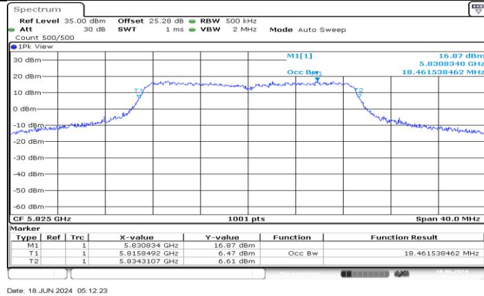
11AC20MIMO_Ant2_5825
