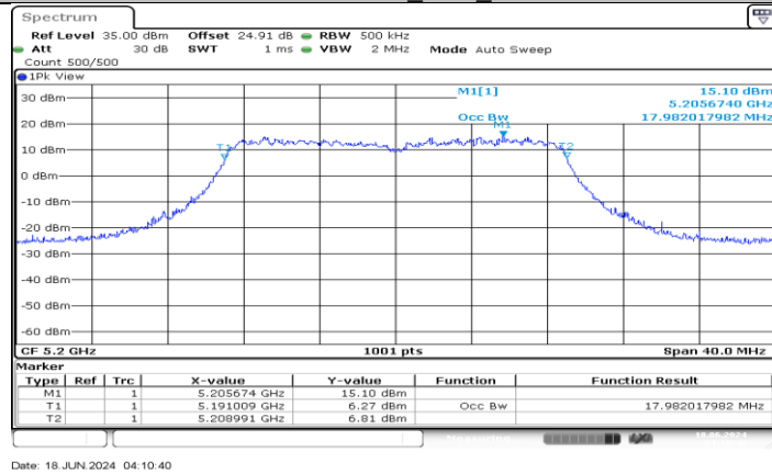
11AC20MIMO_Ant4_5200
