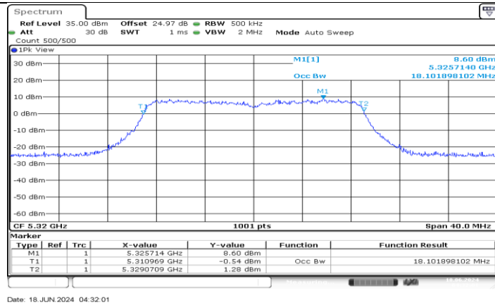
11AC20MIMO_Ant2_5320
