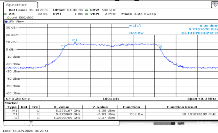
11AC20MIMO_Ant2_5280
