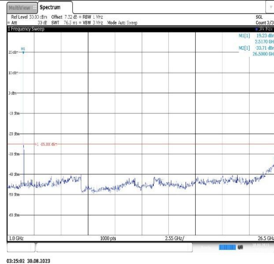
Band7-20MHz-QPSK-21350-1RB#0- Range2:1000~26500MHz
