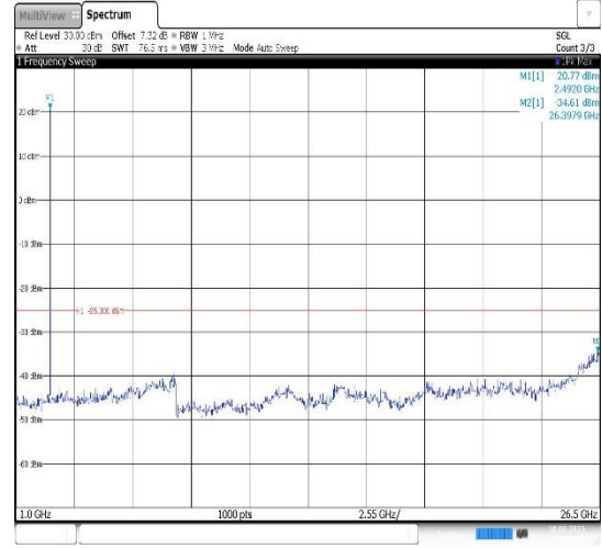
Band7-15MHz-QPSK-20825-1RB#0- Range2:1000~26500MHz
