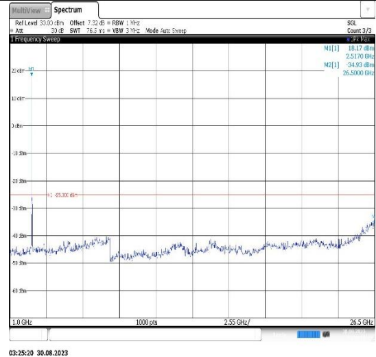
Band7-20MHz-16QAM-21350-1RB#0- Range2:1000~26500MHz
