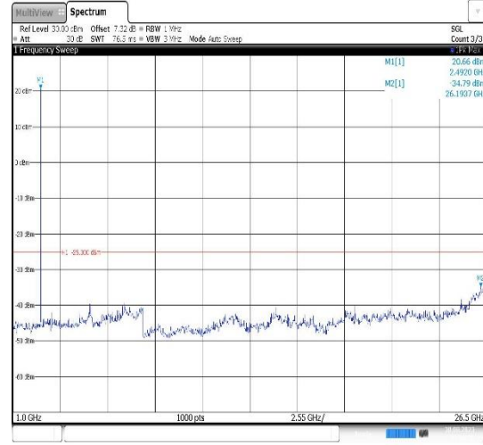
Band7-10MHz-16QAM-20800-1RB#0- Range2:1000~26500MHz
