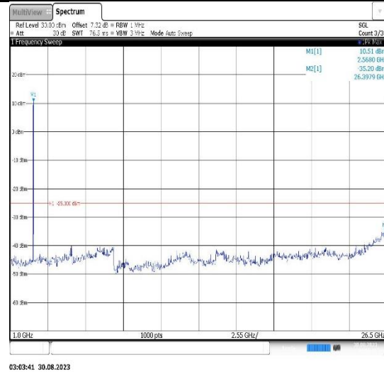
Band7-20MHz-QPSK-20850-1RB#0- Range2:1000~26500MHz
