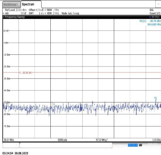
Band7-20MHz-QPSK-21350-1RB#0- Range1:30~1000MHz
