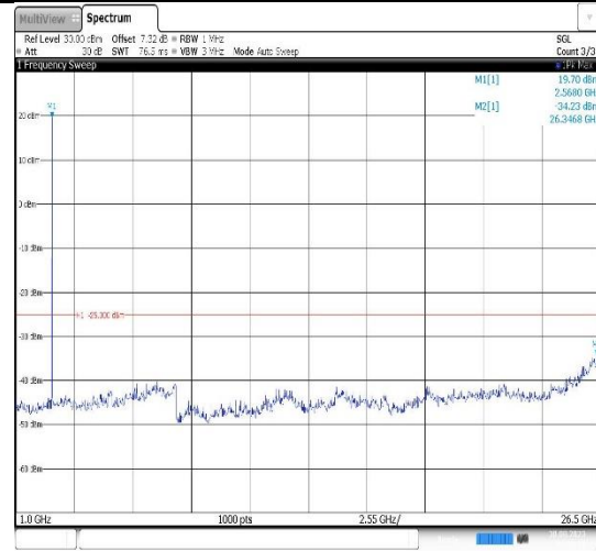
Band7-10MHz-QPSK-20800-1RB#0- Range2:1000~26500MHz
