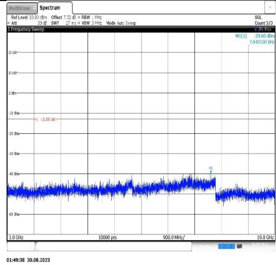
Band5-10MHz-QPSK-20525-1RB#0- Range2:1000~10000MHz
