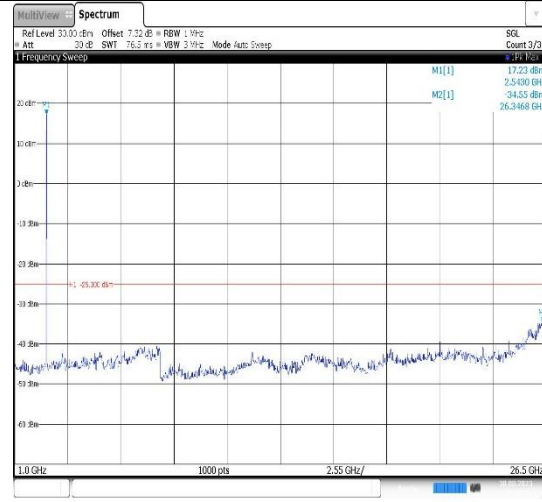
Band7-10MHz-QPSK-21100-1RB#0- Range2:1000~26500MHz
