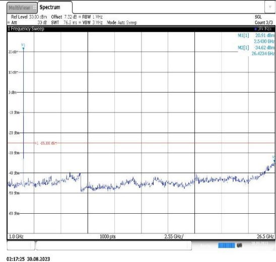
Band7-5MHz-QPSK-21425-1RB#0- Range2:1000~26500MHz
