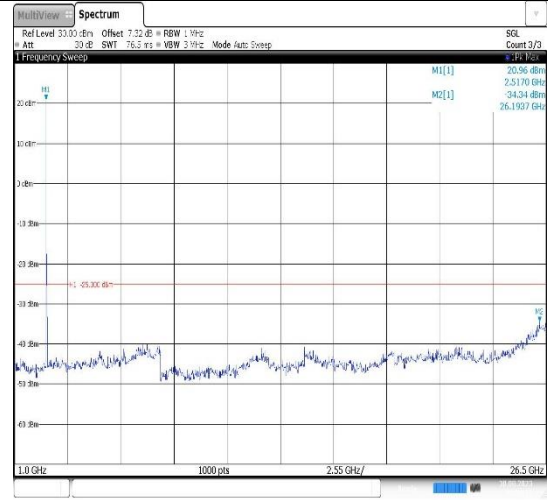
Band7-15MHz-QPSK-21100-1RB#0- Range2:1000~26500MHz
