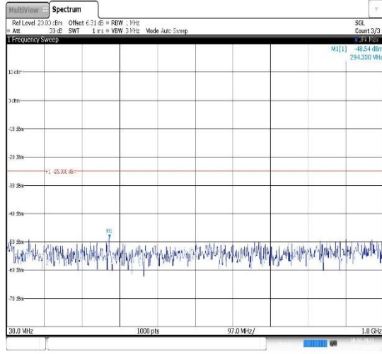
Band7-10MHz-QPSK-20800-1RB#0- Range1:30~1000MHz
