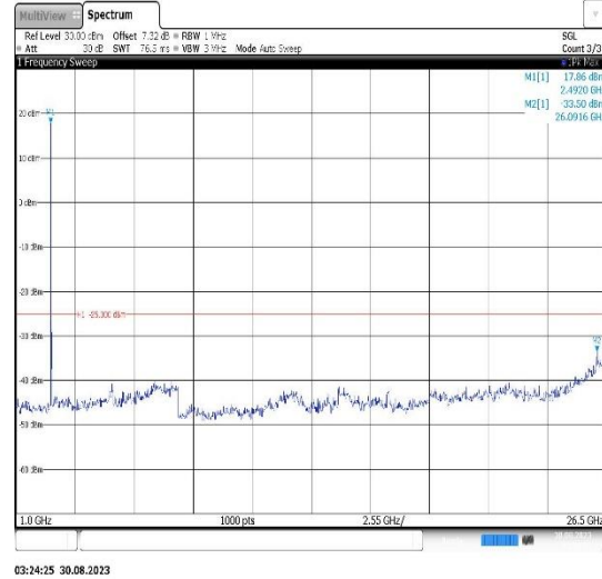
Band7-20MHz-QPSK-21100-1RB#0- Range2:1000~26500MHz
