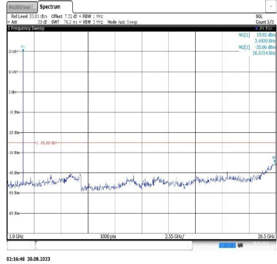
Band7-5MHz-QPSK-21100-1RB#0- Range2:1000~26500MHz
