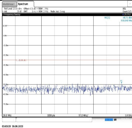
Band7-20MHz-QPSK-20850-1RB#0- Range1:30~1000MHz
