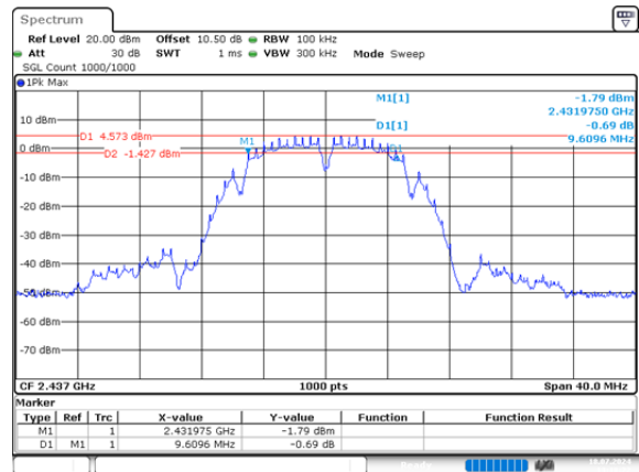
b_2437MHz_Chain 0 9.610MHz
