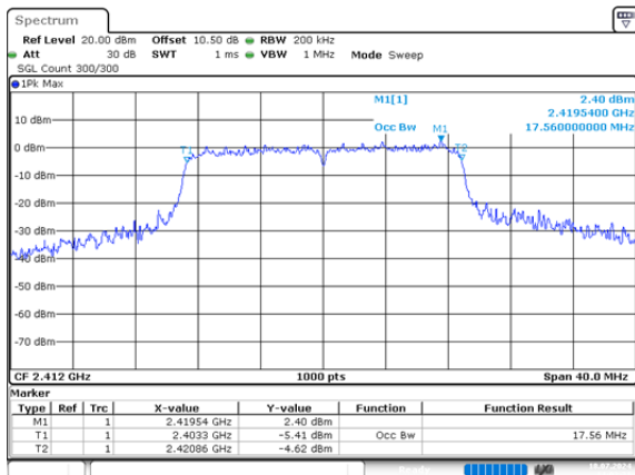
n20_2412MHz_Chain 0 17.560MHz
