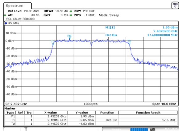
n20_2437MHz_Chain 0 17.600MHz
