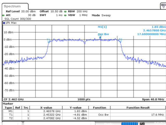
n20_2462MHz_Chain 0 17.600MHz
