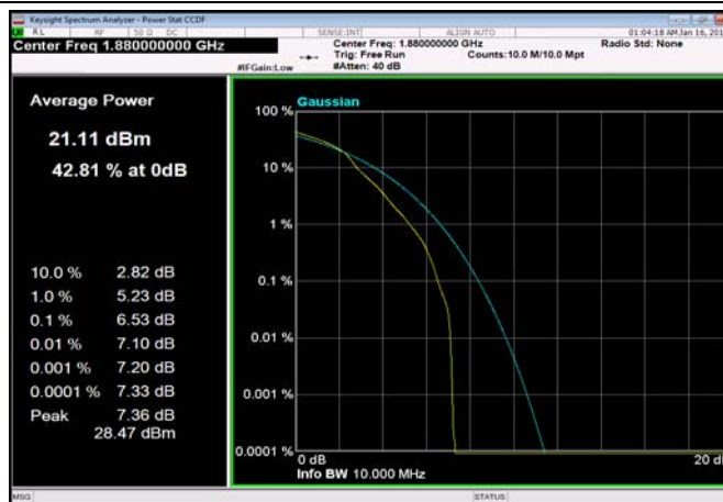
FDD02_10MHz_1880_OneRB_high_Q16
