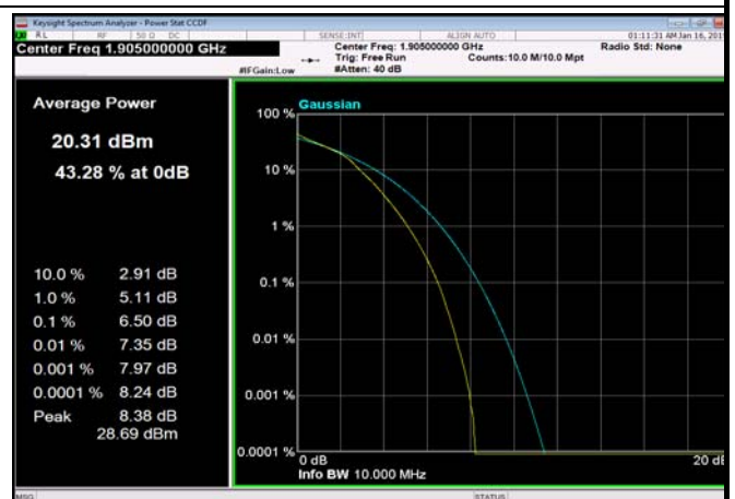
FDD02_10MHz_1905_fullRB_Q16
