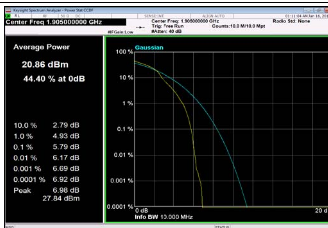
FDD02_10MHz_1905_OneRB_high_Q16
