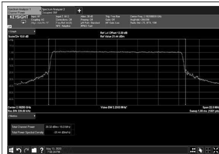
Figure 193: 256QAM 15MHz B.W.; 2192.5MHz, 15kHz
