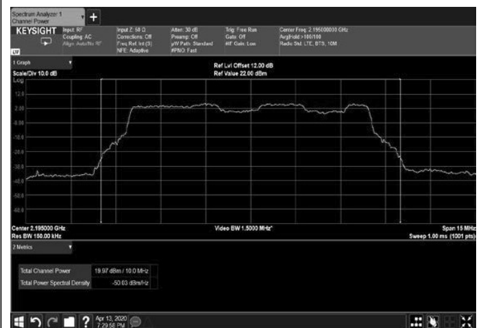
Figure 120: 16QAM 10MHz B.W.; 2195.0MHz, 60kHz
