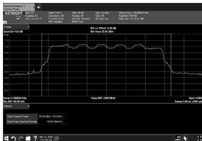
Figure 119: 16QAM 10MHz B.W.; 2195.0MHz, 30kHz
