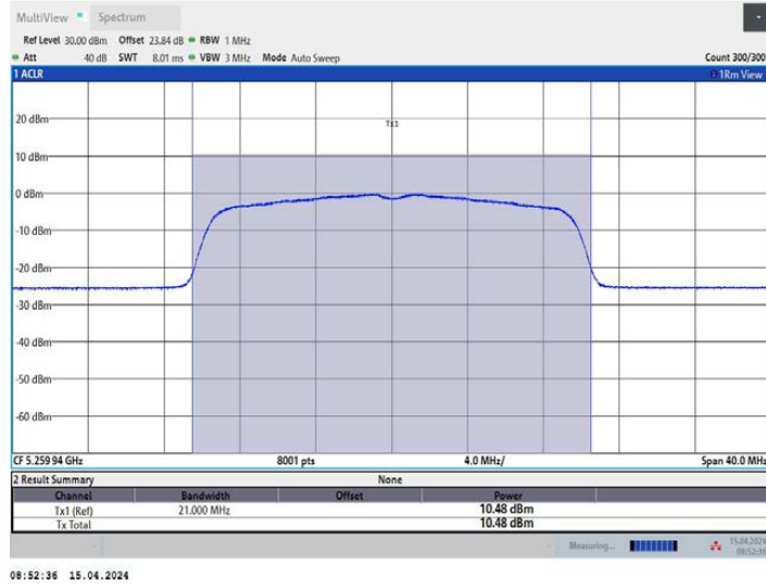
11AX20MIMO_Ant3_5260
