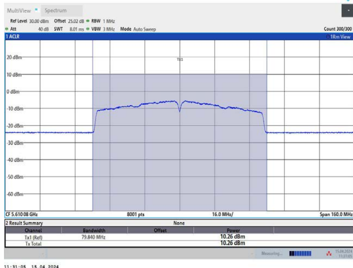
11AC80MIMO_Ant1_5610
