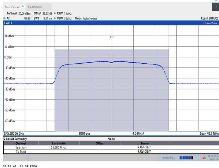
11AX20MIMO_Ant3_5580
