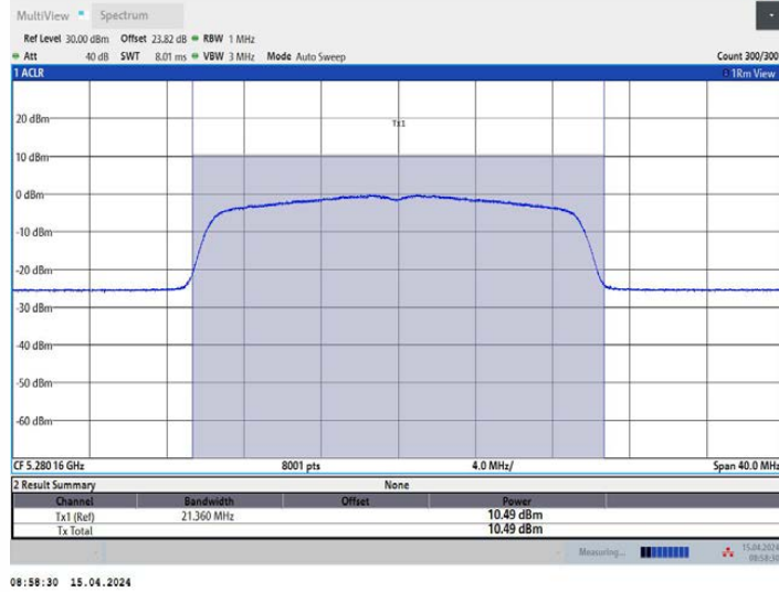
11AX20MIMO_Ant2_5280
