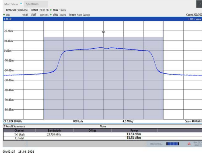
11AC20MIMO_Ant3_5825
