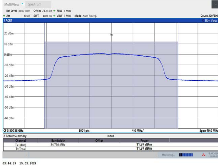
11AX20MIMO_Ant3_5500
