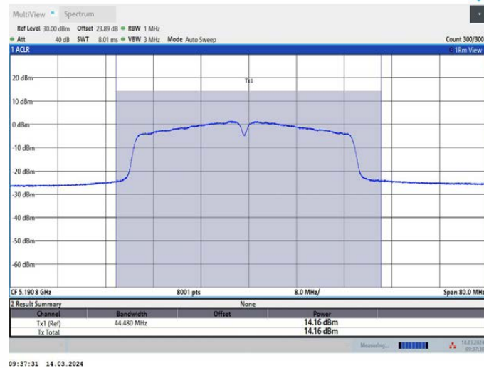
11AC40MIMO_Ant1_5190
