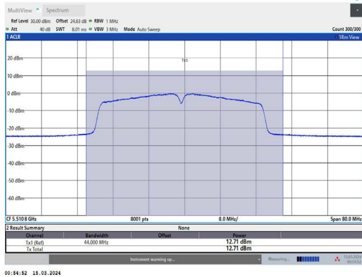
11AC40MIMO_Ant3_5510
