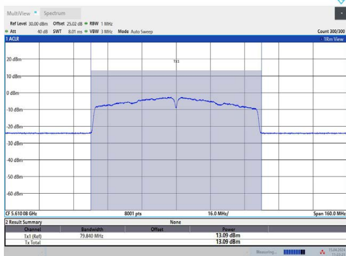
11AC80MIMO_Ant2_5610
