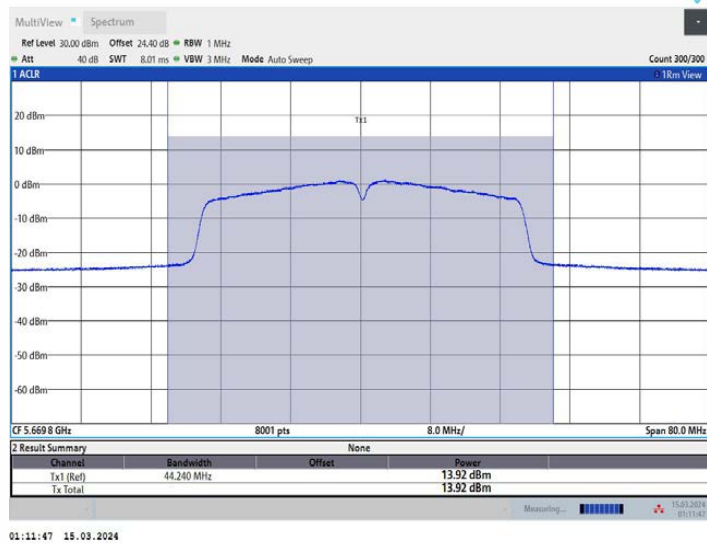
11AC40MIMO_Ant3_5670
