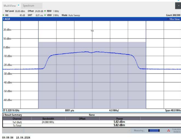
11AX20MIMO_Ant1_5320
