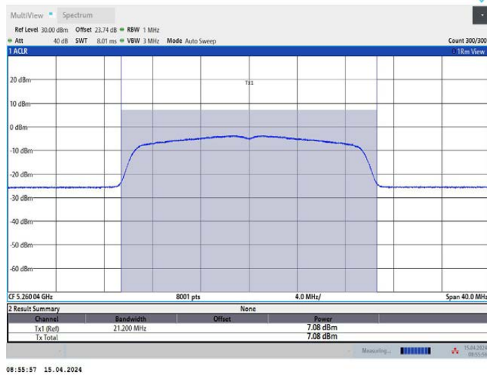
11AX20MIMO_Ant3_5260
