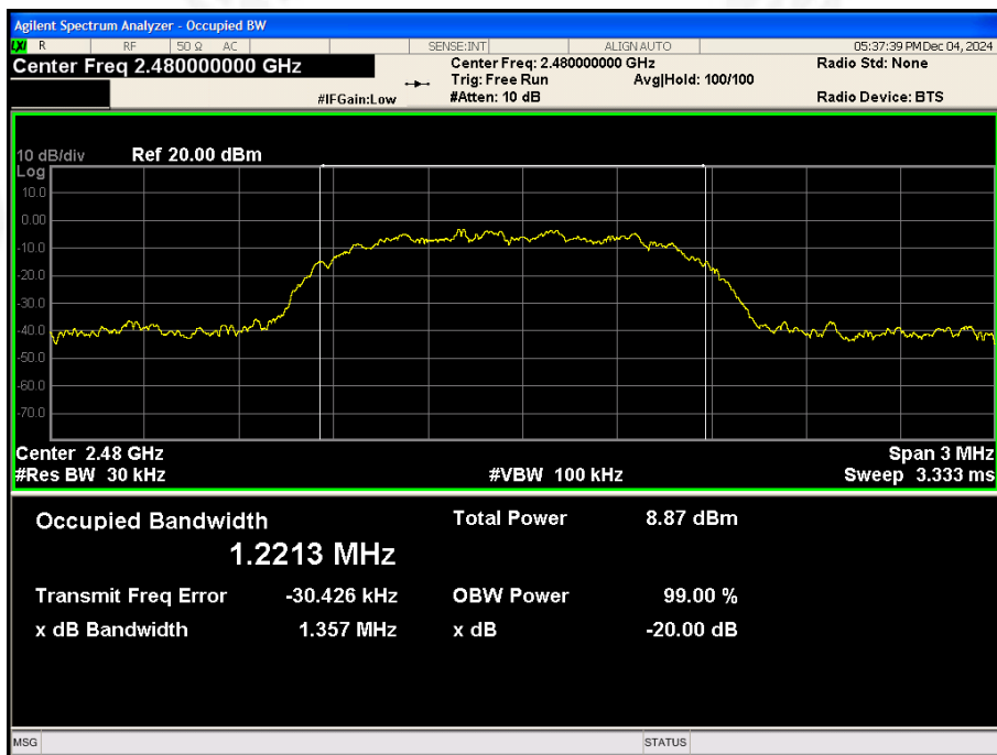
CH78: 2480MHz
