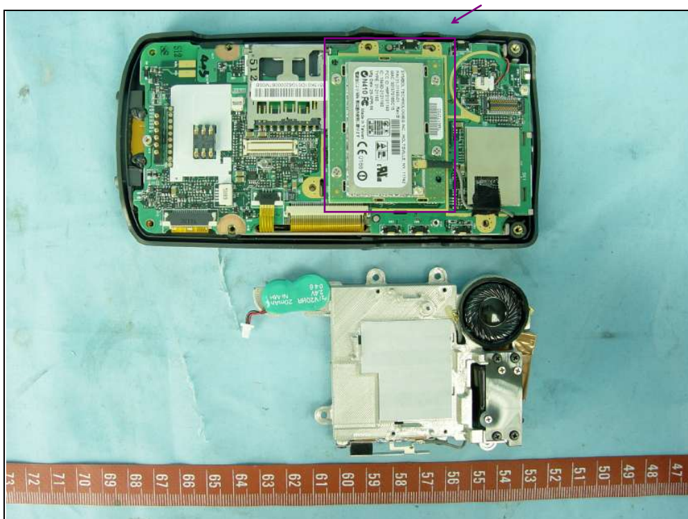
WLAN Module
