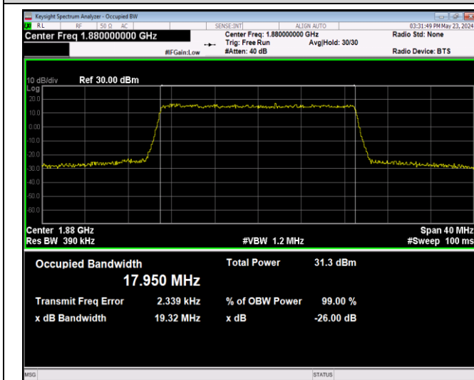
Band2-20MHz-16QAM-18700-100RB#0
