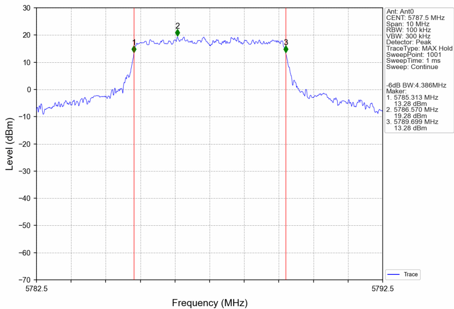
5M_MCH_5787.5MHz_Ant0_NTNV
