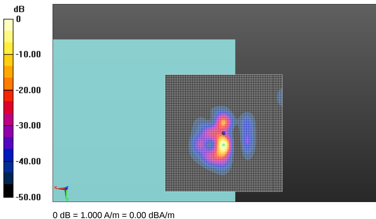
Fig A.35 T-Coil EDGE 850
