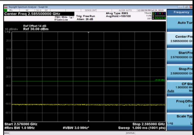
FDD07_20MHz_2510_Q16_fullRB_ExtraBand s_Range_2576~2595
