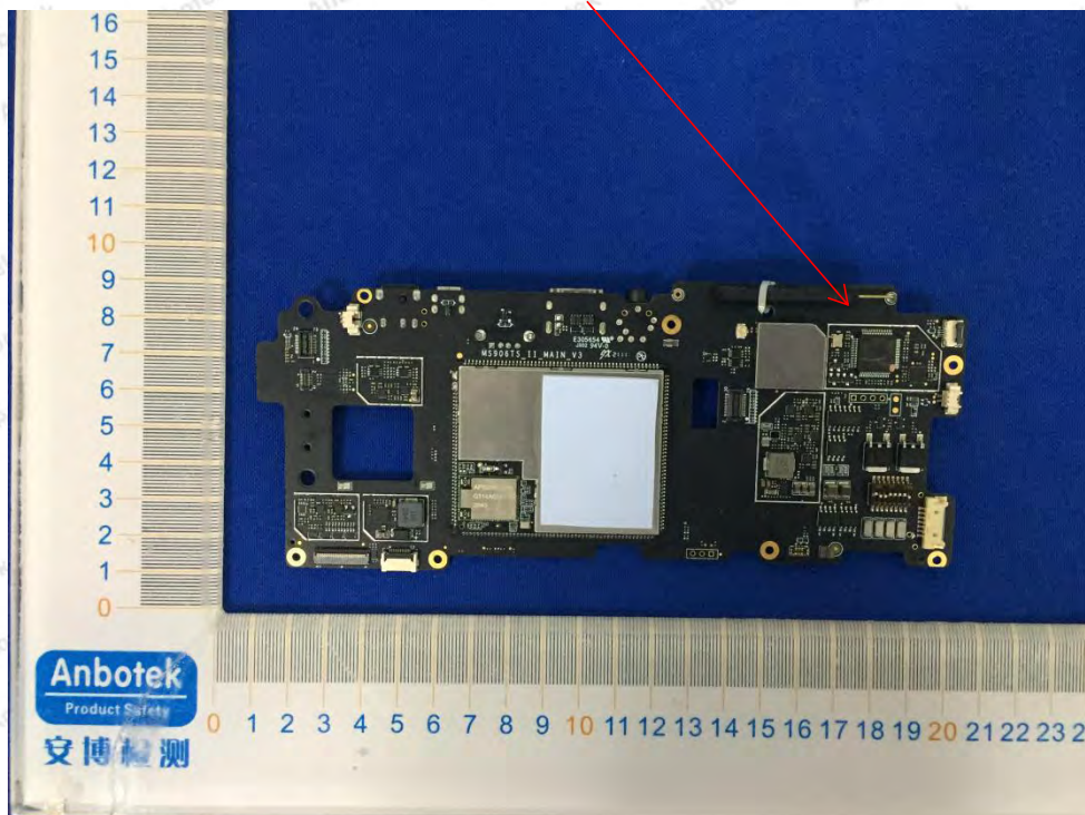
315MHz&433.92MHz&125KHz ANT
