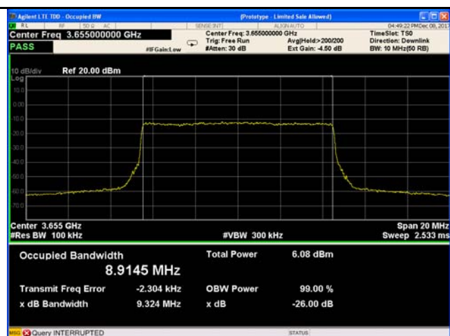
10MHz - Low CH 16QAM
