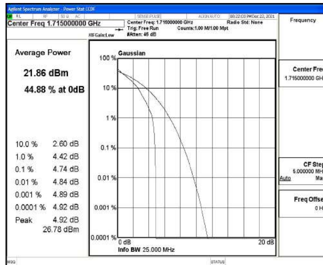
Band4-10MHz-QPSK-20000-50RB#0
