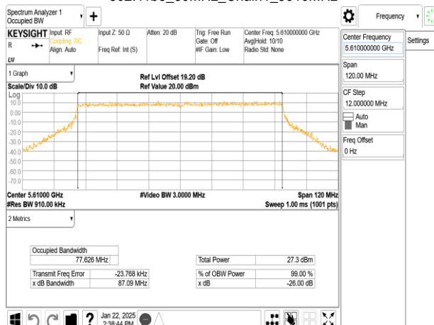
802.11be_80MHz_Chain1_5610MHz
