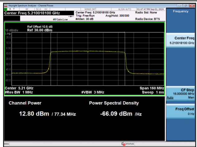
11AX80MIMO-Ant1-5210-PASS
