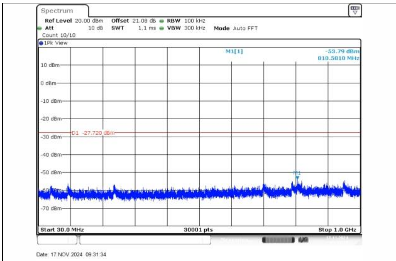
11G-Ant1-2462-30~1000-PASS
