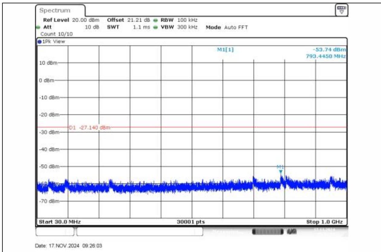
11G-Ant1-2412-30~1000-PASS
