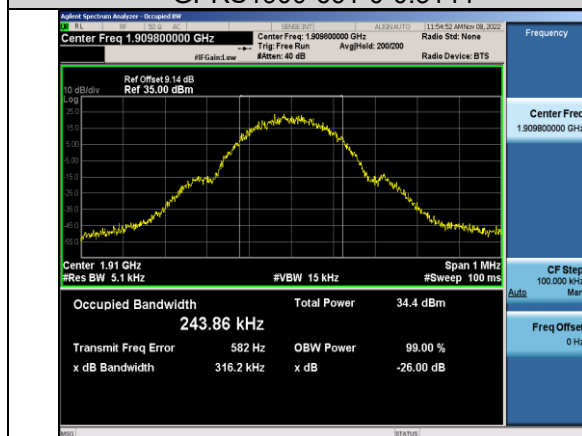
GPRS1900-810-0-0.3162
