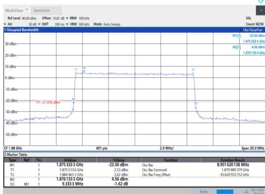
Band2-10MHz-16QAM-18900-50RB#0
