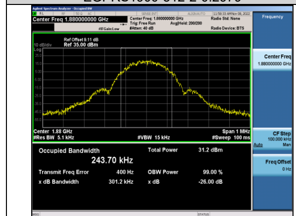
EGPRS1900-661-2-0.3012
