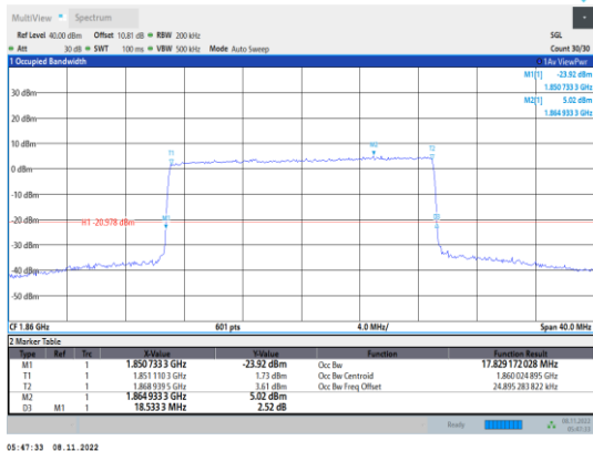
Band2-20MHz-16QAM-18700-100RB#0
