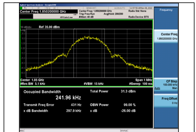
EGPRS1900-512-2-0.2979
