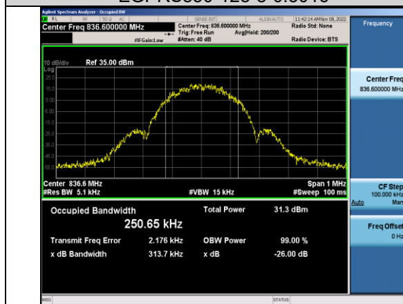
EGPRS850-190-8-0.3137
