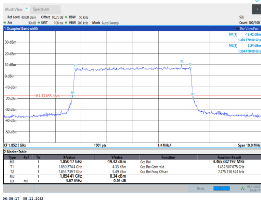
Band2-5MHz-QPSK-18625-25RB#0
