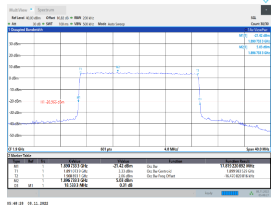
Band2-20MHz-QPSK-19100-100RB#0
