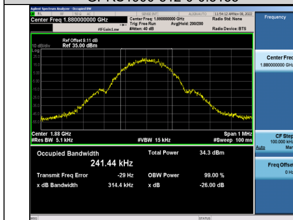
GPRS1900-661-0-0.3144
