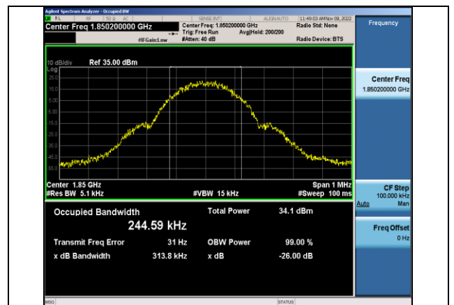
GSM1900-512-0-0.3138
