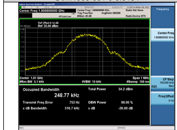
GSM1900-810-0-0.3167
