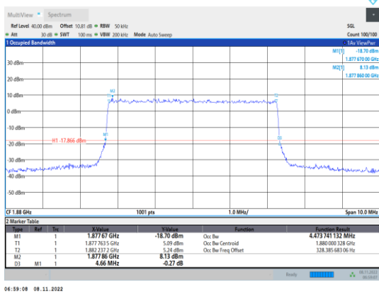
Band2-5MHz-QPSK-18900-25RB#0
