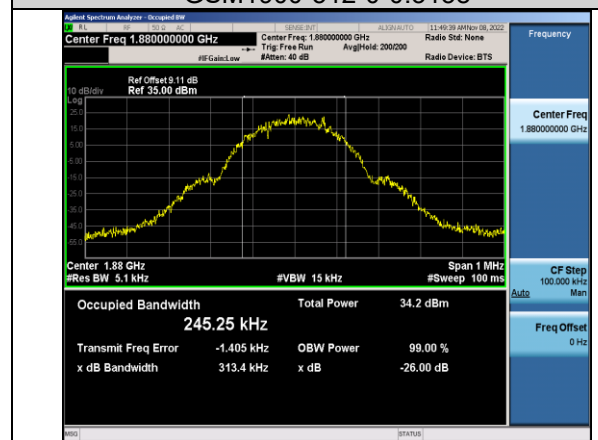
GSM1900-661-0-0.3134
