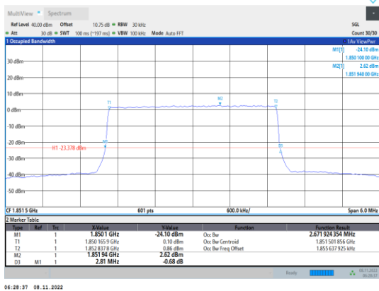
Band2-3MHz-16QAM-18615-15RB#0
