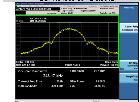
EGPRS1900-810-2-0.3093
