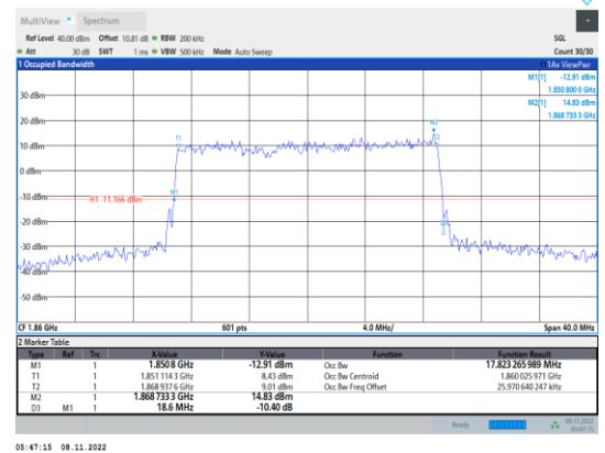
Band2-20MHz-QPSK-18700-100RB#0
