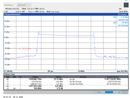
Band2-20MHz-QPSK-18900-100RB#0
