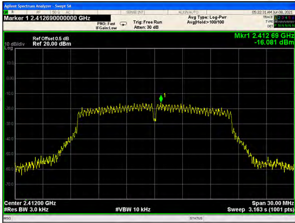
CH1: 2412MHz-ANT1
