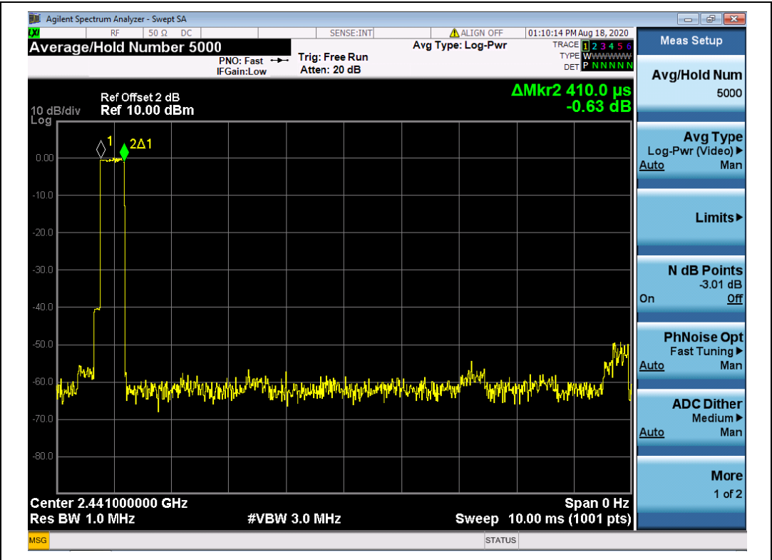
(DH1, 8-DPSK)
