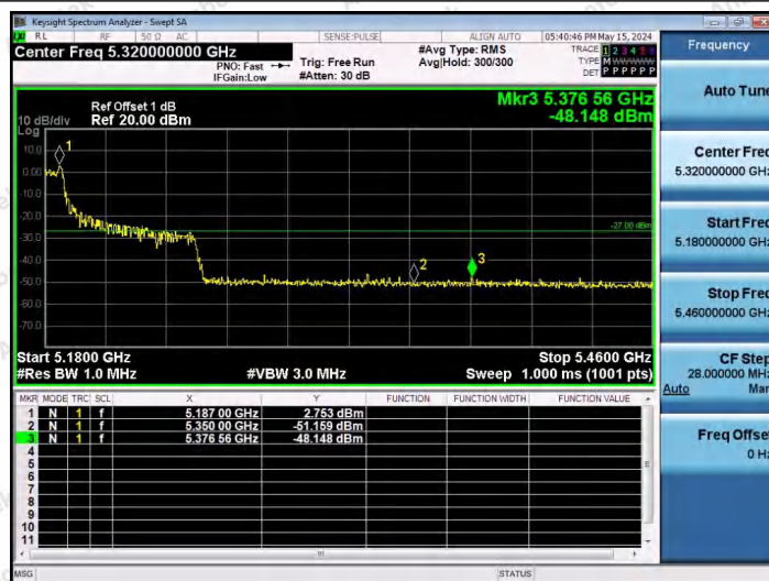
11AX80SISO-Ant1-5210-52Tone-RU37-PASS
