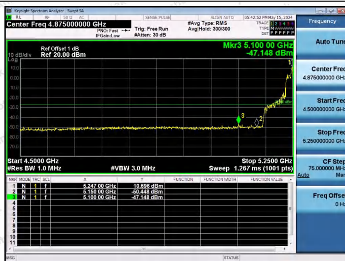
11AX80SISO-Ant1-5210-52Tone-RU52-PASS
