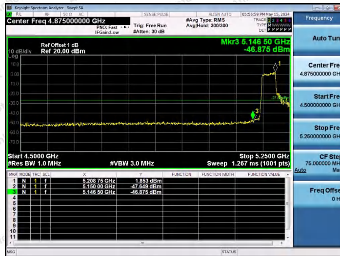
11AX80SISO-Ant1-5210-484Tone-RU65-PASS
