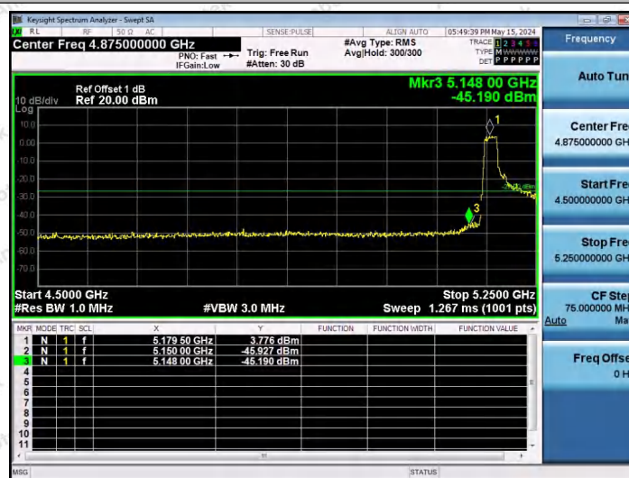
11AX80SISO-Ant1-5210-242Tone-RU61-PASS
