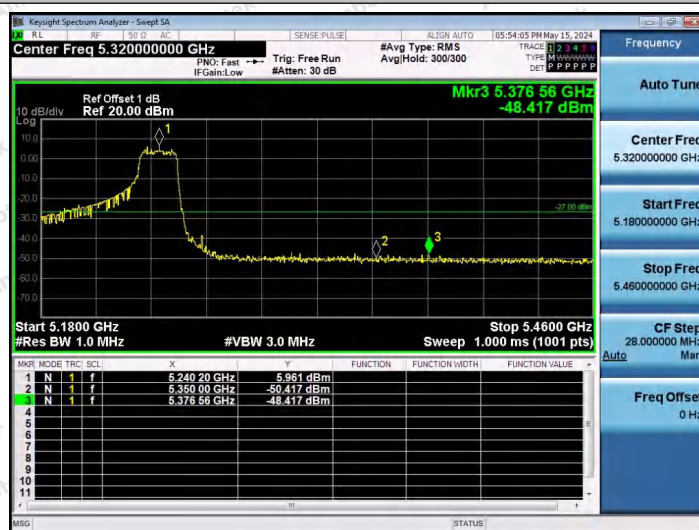
11AX80SISO-Ant1-5210-242Tone-RU64-PASS
