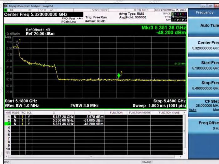
11AX80SISO-Ant1-5210-242Tone-RU61-PASS
