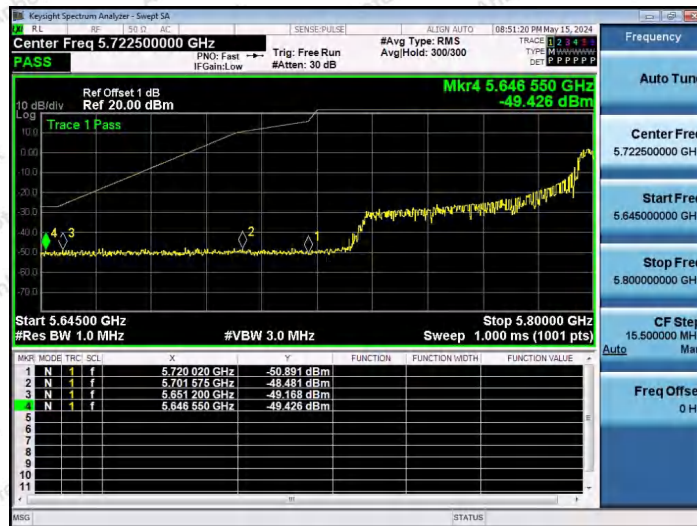
11AX80SISO-Ant1-5775-52Tone-RU52-PASS
