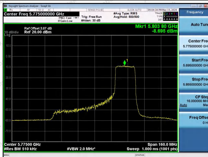
11AX80SISO-Ant1-5775-242Tone-RU64-PASS
