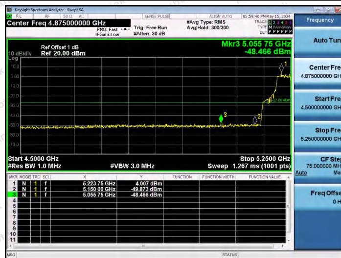
11AX80SISO-Ant1-5210-484Tone-RU66-PASS
