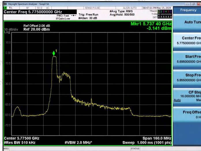
11AX80SISO-Ant1-5775-52Tone-RU37-PASS
