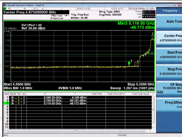
11AX80SISO-Ant1-5210-242Tone-RU64-PASS
