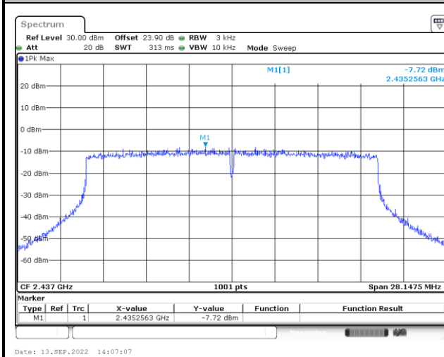
MIMO Ant. 0
