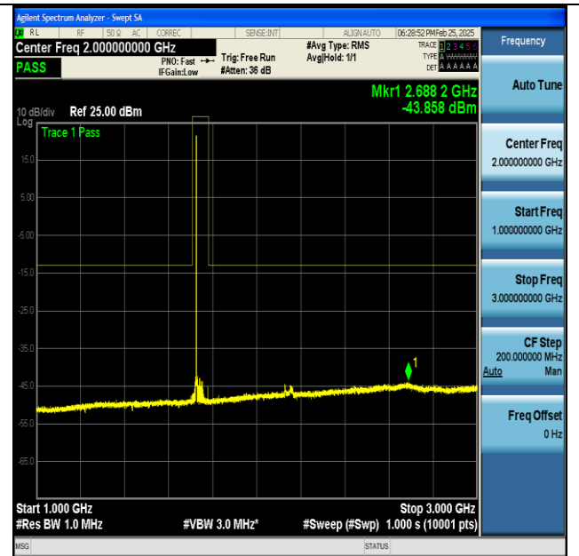
NTNV-n66-PC3-15-40-M-CP-QPSK-Edge_1RB_Left-1000-3000-PASS
