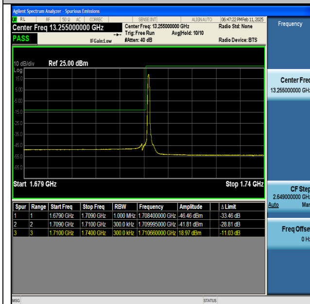
NTNV-n66-PC3-15-30-L-CP-QPSK-Edge_1RB_Left-PASS
