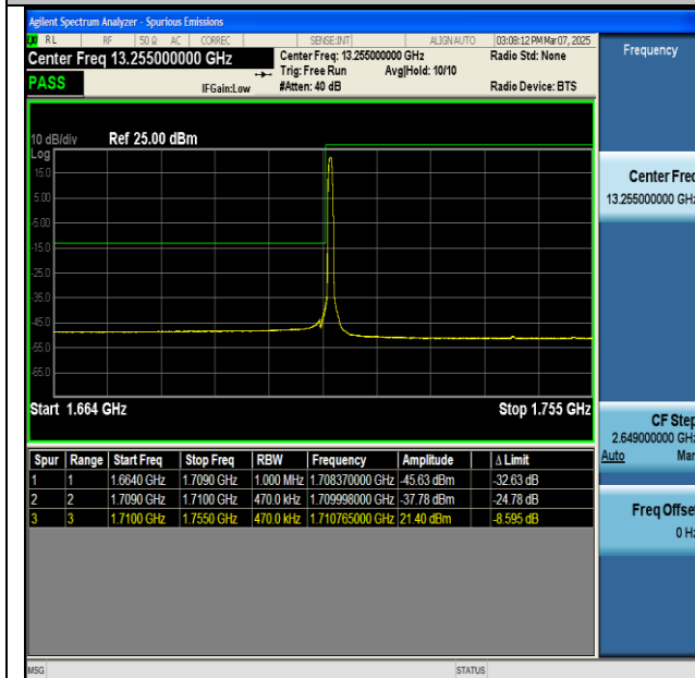
NTNV-n66-PC3-15-45-L-CP-QPSK-Edge_1RB_Left-PASS
