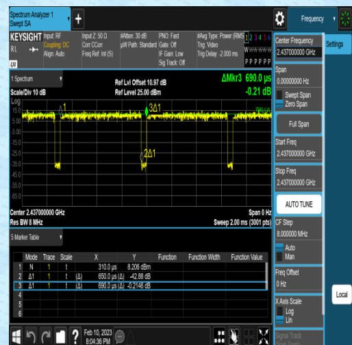
NTNV-11N40MIMO-Ant2-2437
