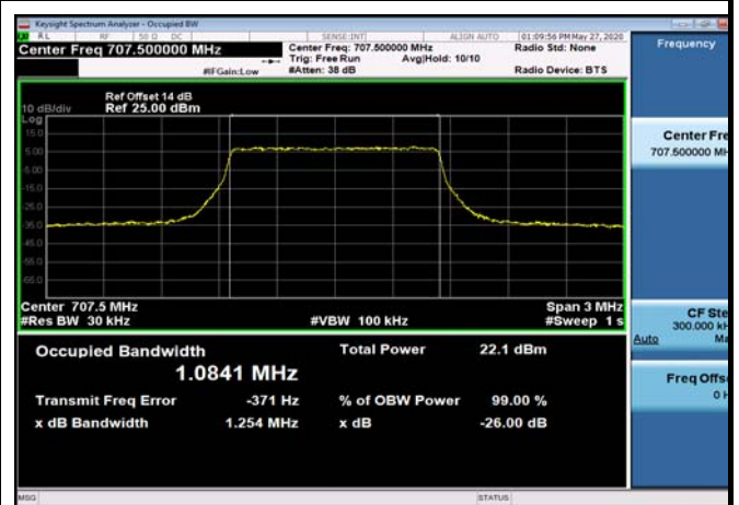
FDD12_MidRange_3_707.5_Q16
