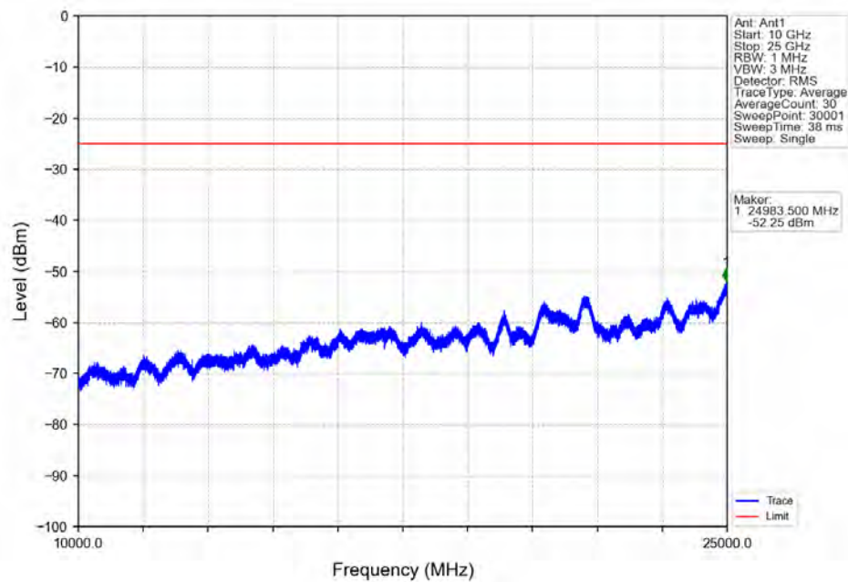
Band7_20MHz_16QAM_MCH_2535MHz_RB_1_0_NTV
