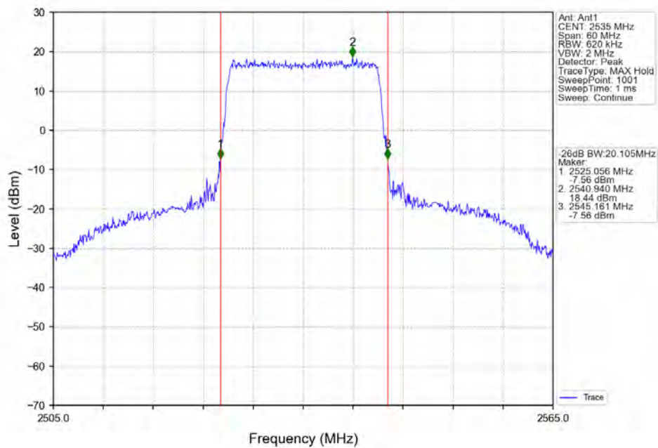
Band7_20MHz_16QAM_MCH_2535MHz_RB_100_0_NTNV
