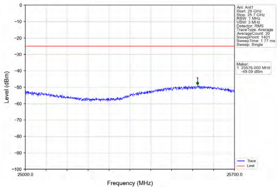
Band7_5MHz_QPSK_MCH_2535MHz_RB_1_0_NTN
