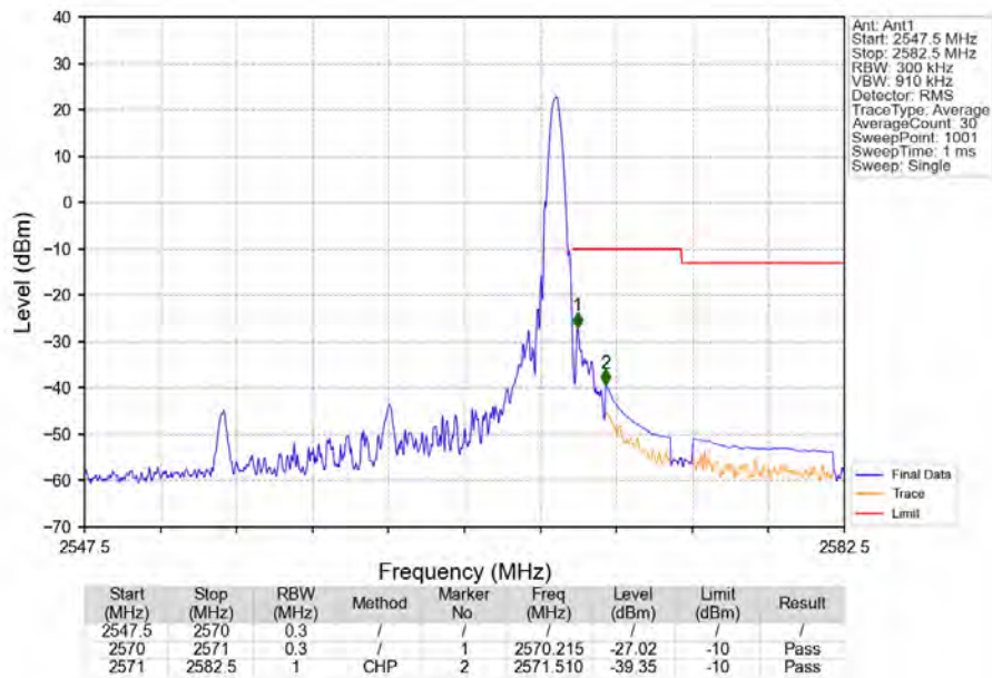
Band7_15MHz_QPSK_HCH_2562.5MHz_RB_1_74_NTV
