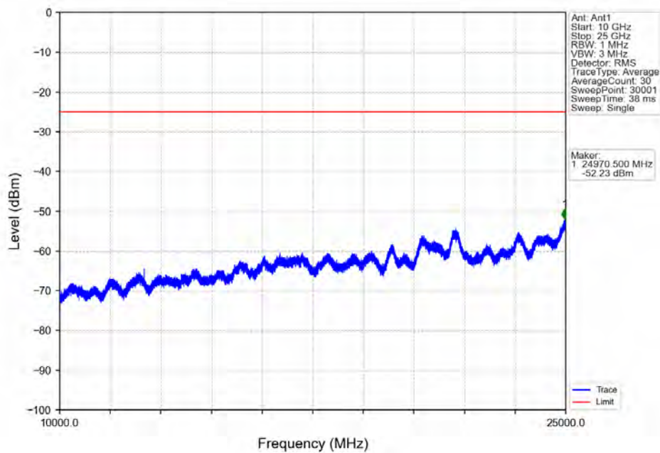
Band7_20MHz_16QAM_LCH_2510MHz_RB_1_0_NTNV
