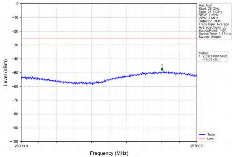
Band7_15MHz_QPSK_HCH_2562.5MHz_RB_1_74_NTV
