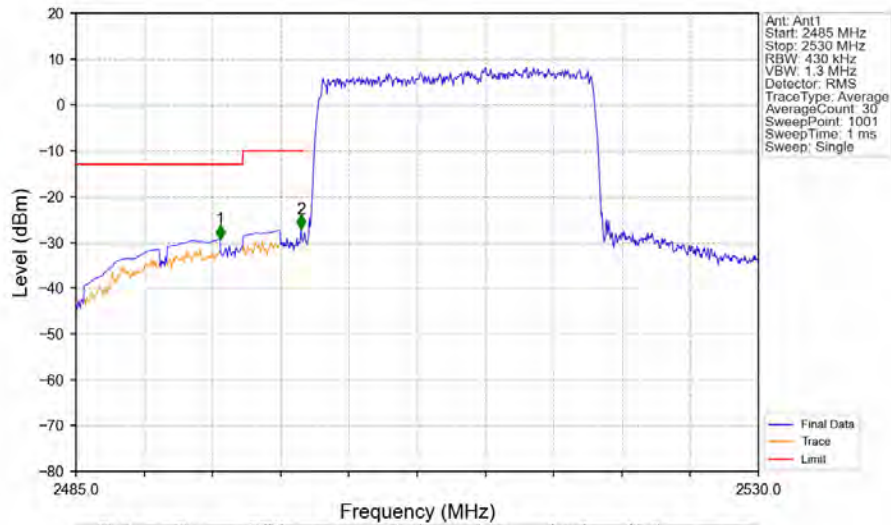
Band7_20MHz_16QAM_LCH_2510MHz_RB_100_0_NTNV
