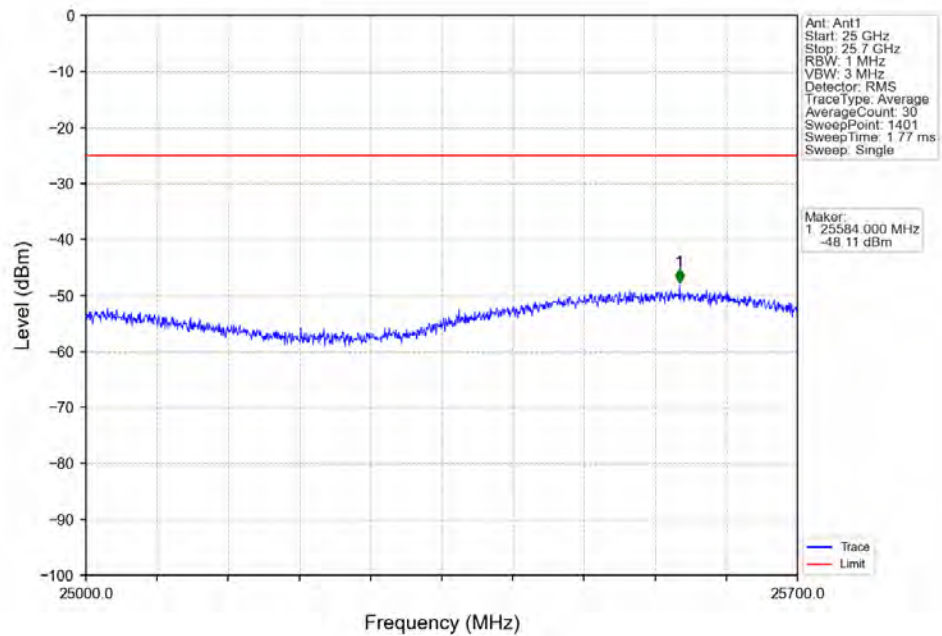
Band7_20MHz_64QAM_MCH_2535MHz_RB_1_0_NTNV
