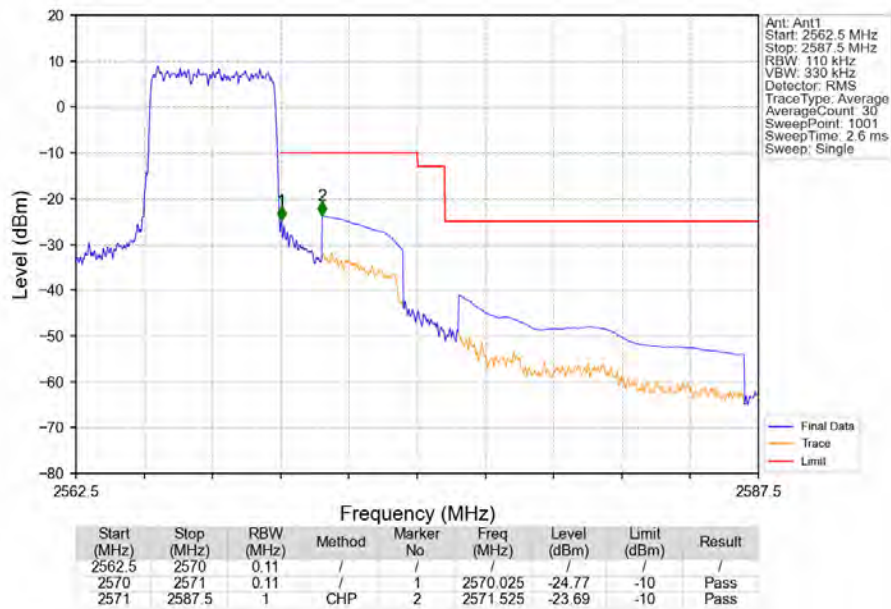
Band7 5MHz QPSK HCH 2567.5MHz RB 25 0 NTV
