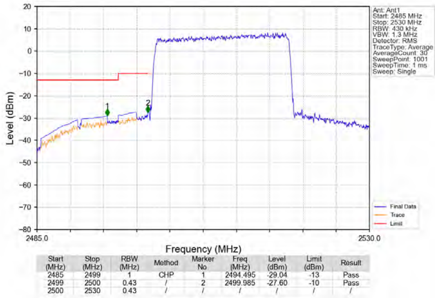
Band7 20MHz 64QAM LCH 2510MHz RB 100 0 NTNV
