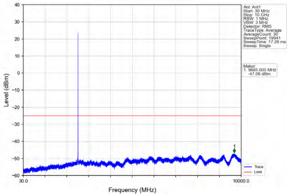
Band7_5MHz_QPSK_MCH_2535MHz_RB_1_0_NTN
