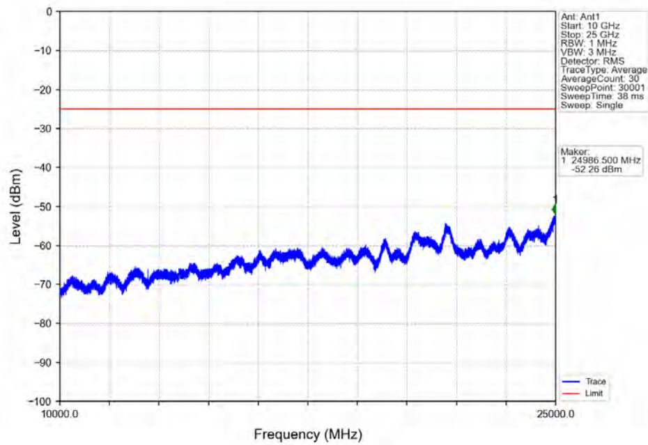
Band7_5MHz_QPSK_MCH_2535MHz_RB_1_0_NTN
