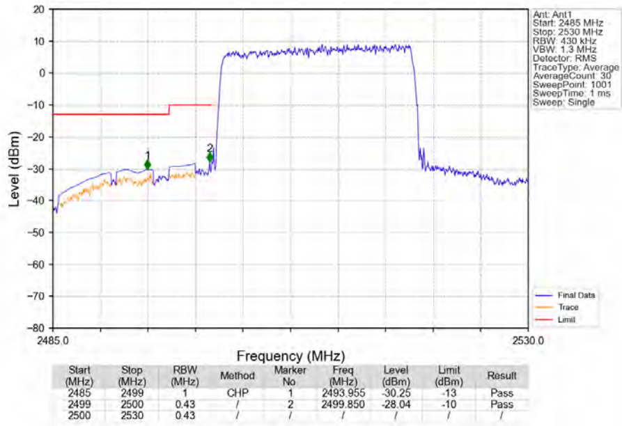
Band7 20MHz QPSK LCH 2510MHz RB 100 0 NTNV
