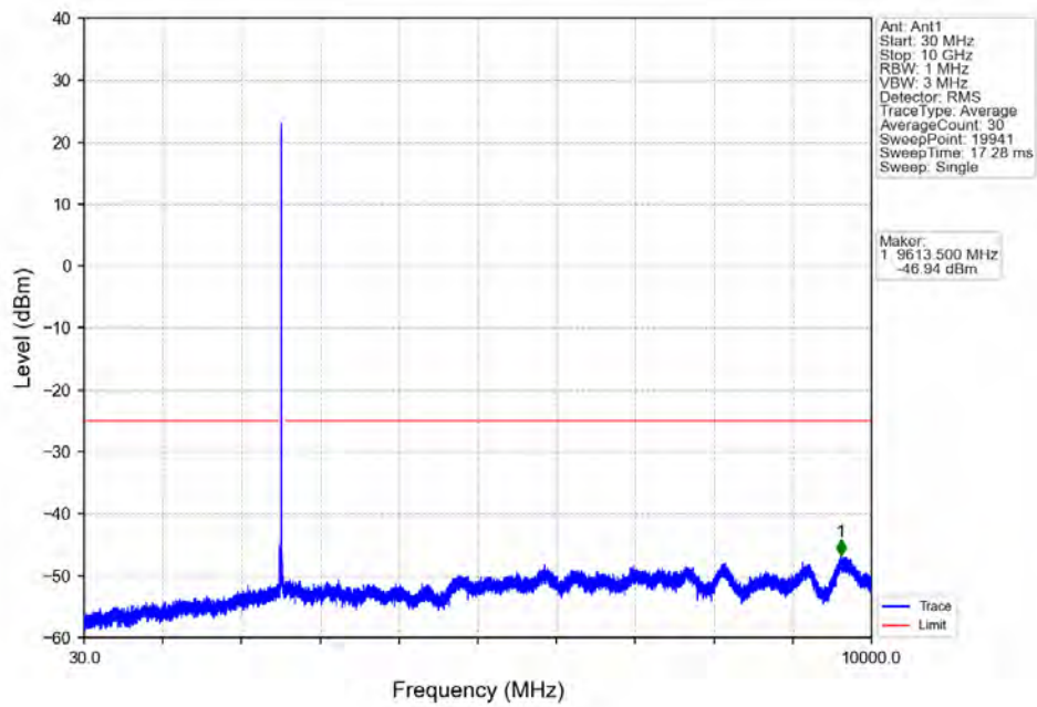
Band7_20MHz_16QAM_MCH_2535MHz_RB_1_0_NTV
