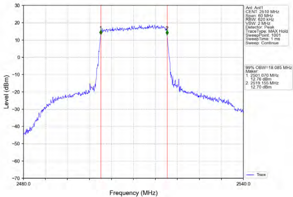
Band7_20MHz_64QAM_LCH_2510MHz_RB_100_0_NTNV
