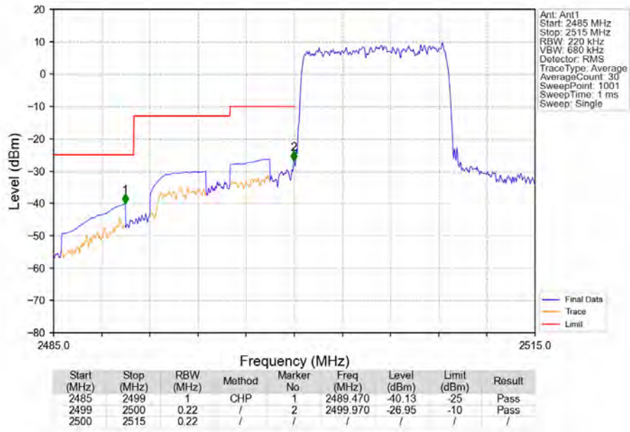
Band7 10MHz QPSK LCH 2505MHz RB 50 0 NTNV
