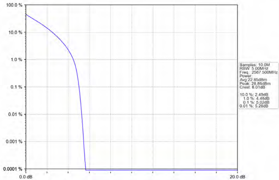
Band7 5MHz QPSK HCH 2567.5MHz RB 25 0 NTV
