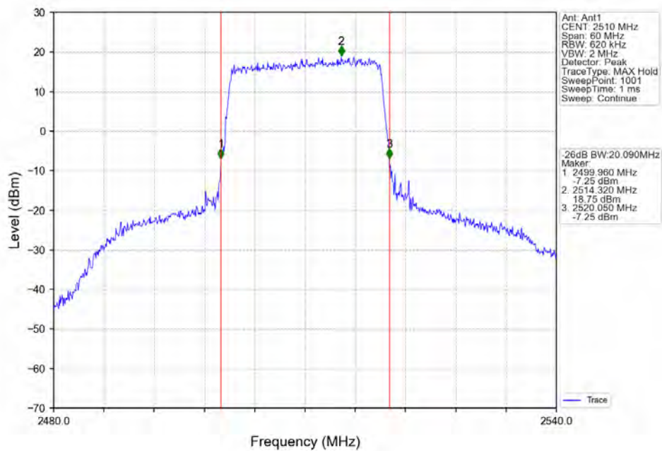
Band7_20MHz_64QAM_LCH_2510MHz_RB_100_0_NTNV
