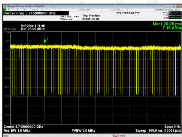
802.11a
