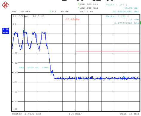
DH1_Hopping_Upper
