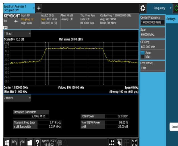
Band2-3MHz-16QAM-18615-15RB#0
