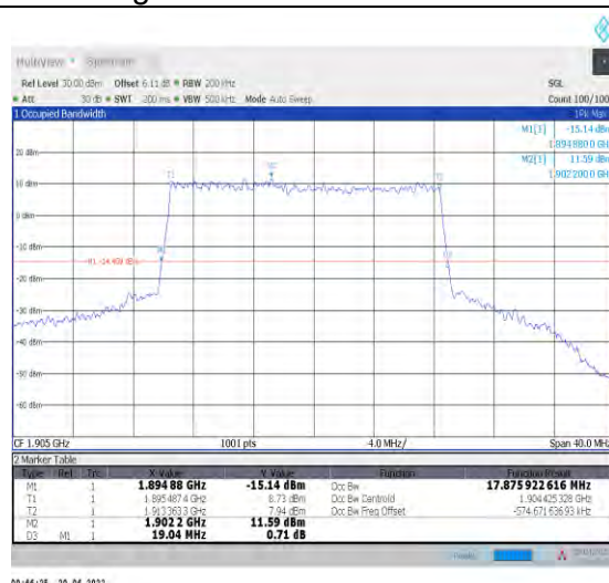
1-N25--15-20-H-3-DFT-16QAM-Outet_Full-100@0-A nt0-17.876-19.040-≤20-PASS
