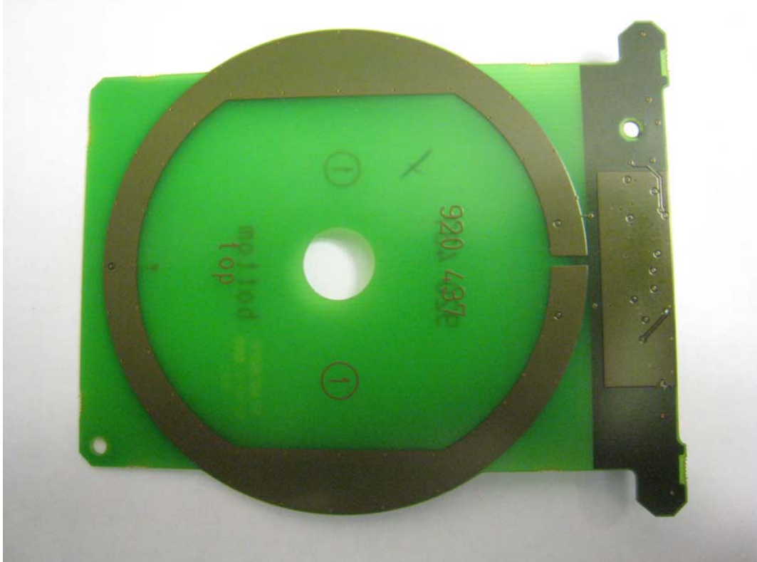
(10) EUT Photo
