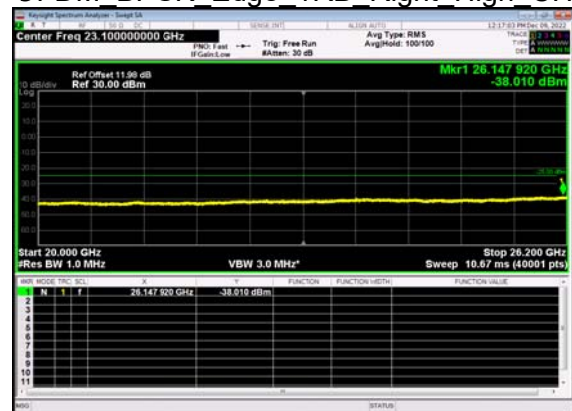
N38(20M)_DFT-s- OFDM BPSK Edge 1RB Right High CH
