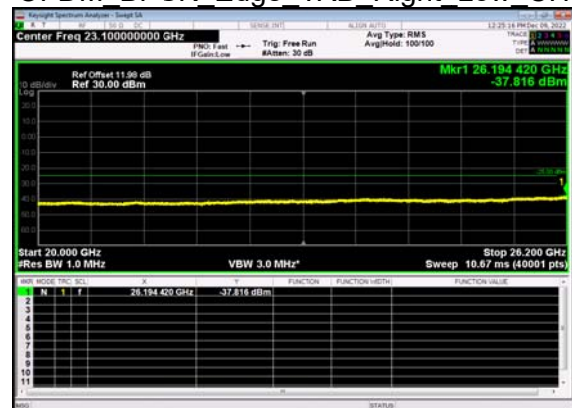
N38(40M)_DFT-s- OFDM BPSK Edge 1RB Right Low CH
