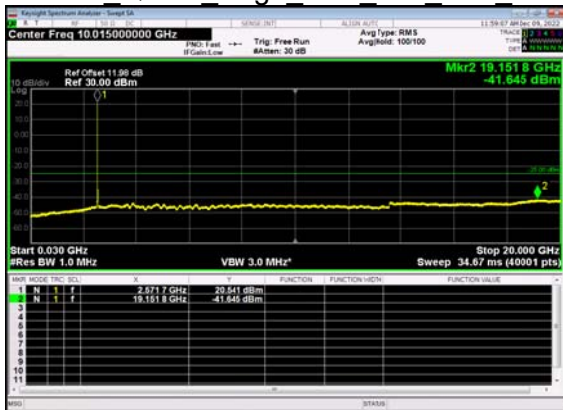
N38(20M)_DFT-s- OFDM QPSK Edge 1RB Left Low CH
