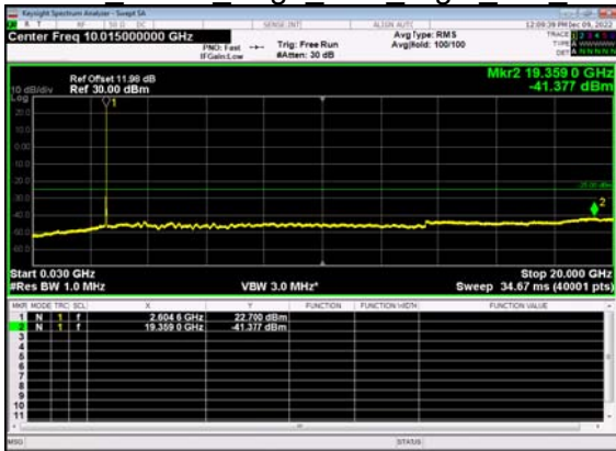
N38(20M)_DFT-s- OFDM QPSK Edge 1RB Right Mid CH
