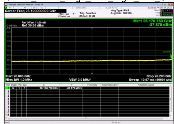
N38(20M)_DFT-s- OFDM BPSK Edge 1RB Right Low CH
