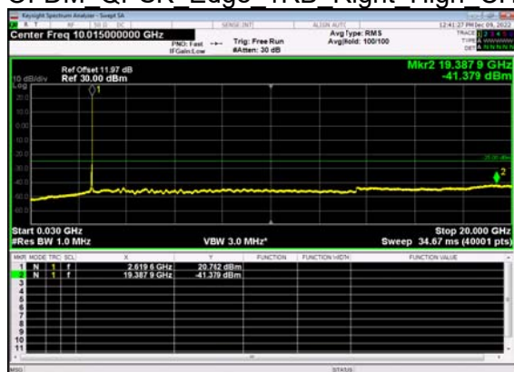
N38(40M)_DFT-s- OFDM QPSK Edge 1RB Right High CH
