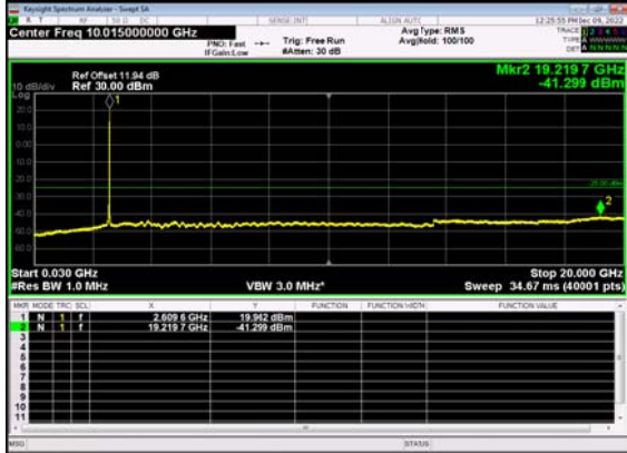
N38(40M)_DFT-s- OFDM QPSK Edge 1RB Right Low CH
