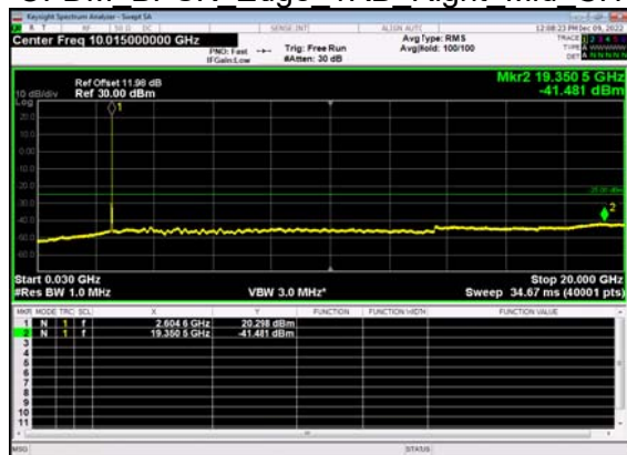
N38(20M)_DFT-s- OFDM BPSK Edge 1RB Right Mid CH
