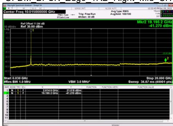
N38(40M)_DFT-s- OFDM BPSK Edge 1RB Right Mid CH
