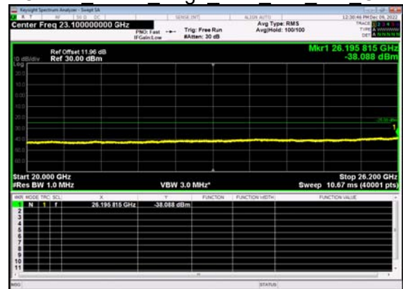
N38(40M)_DFT-s- OFDM BPSK Edge 1RB Left Mid CH
