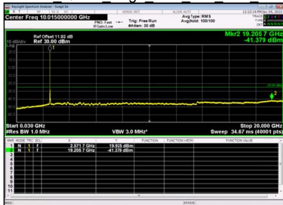
N38(40M)_DFT-s- OFDM QPSK Edge 1RB Left Low CH
