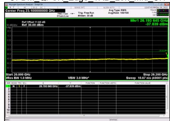
N38(20M)_DFT-s- OFDM QPSK Edge 1RB Left Mid CH
