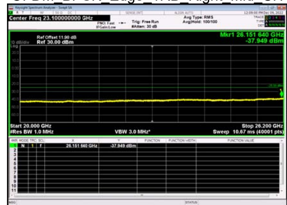
N38(20M)_DFT-s- OFDM BPSK Edge 1RB Right Mid CH
