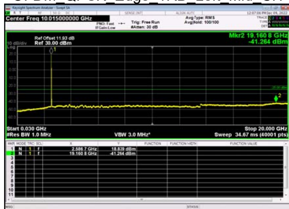
N38(20M)_DFT-s- OFDM QPSK Edge 1RB Left Mid CH
