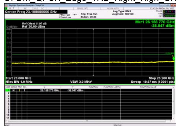
N38(40M)_DFT-s- OFDM QPSK Edge 1RB Right High CH
