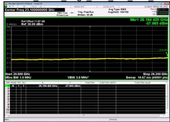
N38(20M)_DFT-s- OFDM BPSK Edge 1RB Left Low CH
