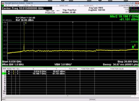
N38(40M)_DFT-s- OFDM QPSK Edge 1RB Right Mid CH
