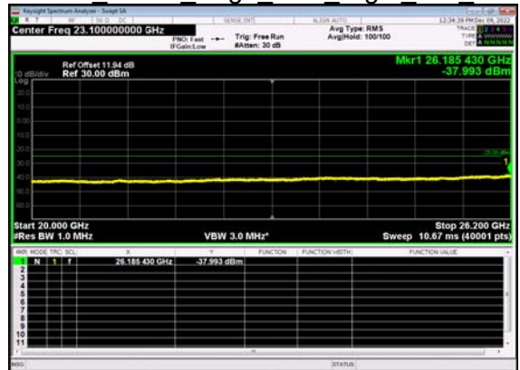
N38(40M)_DFT-s- OFDM QPSK Edge 1RB Right Mid CH
