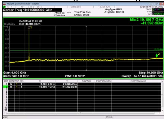
N38(20M)_DFT-s- OFDM QPSK Edge 1RB Left High CH
