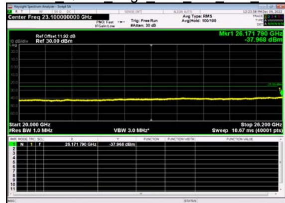
N38(40M)_DFT-s- OFDM QPSK Edge 1RB Left Low CH
