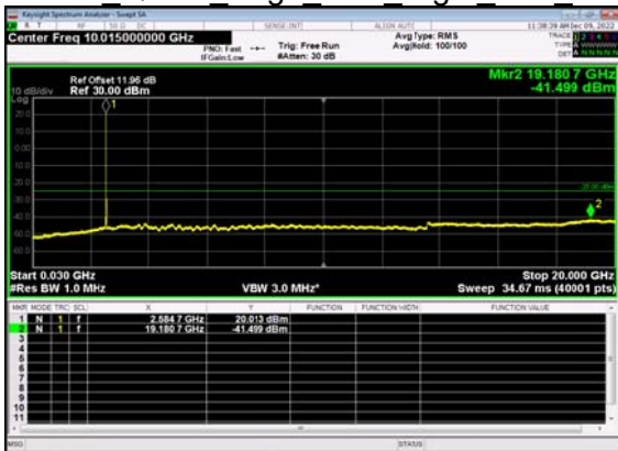
N38(15M)_DFT-s- OFDM QPSK Edge 1RB Right Low CH
