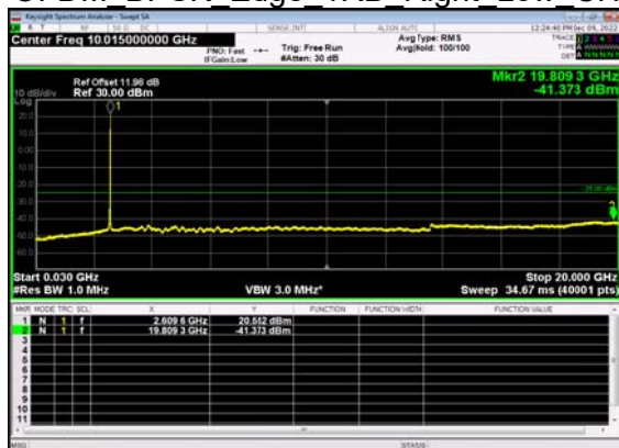
N38(40M)_DFT-s- OFDM BPSK Edge 1RB Right Low CH
