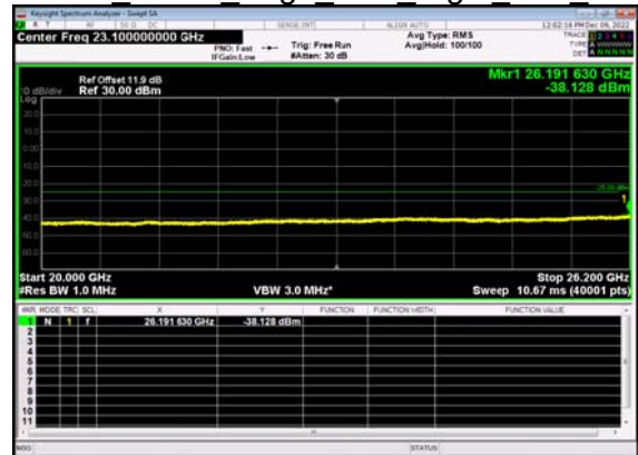
N38(20M)_DFT-s- OFDM QPSK Edge 1RB Right Low CH
