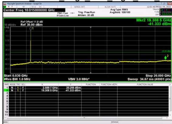
N38(20M)_DFT-s- OFDM QPSK Edge 1RB Right Low CH
