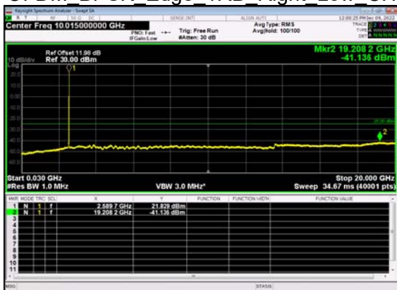
N38(20M)_DFT-s- OFDM BPSK Edge 1RB Right Low CH
