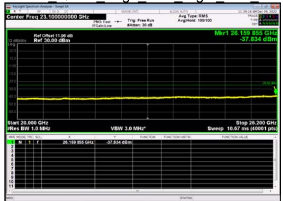
N38(15M)_DFT-s- OFDM QPSK Edge 1RB Right Low CH
