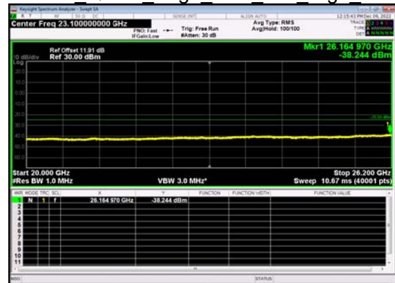
N38(20M)_DFT-s- OFDM QPSK Edge 1RB Left High CH
