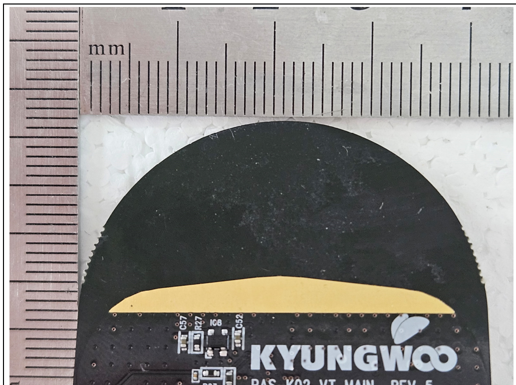
<UWB Antenna >
