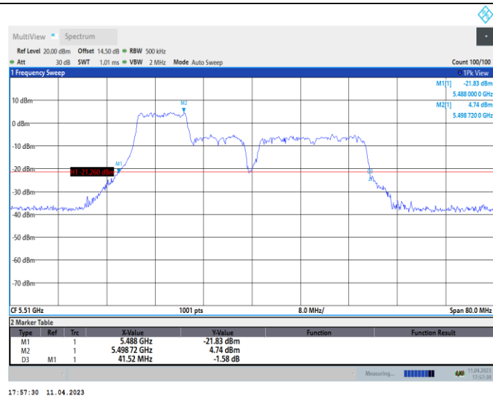
11AX40 Ant9 5510 242Tone RU61
