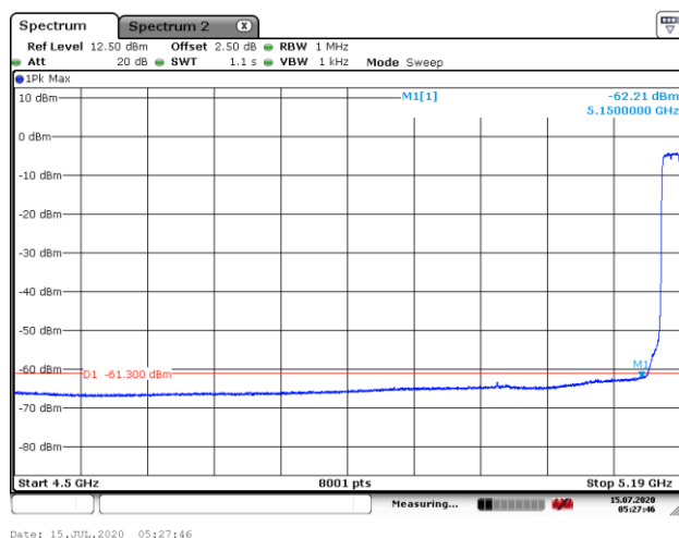
5200MHz with 4*4 CDD AV
