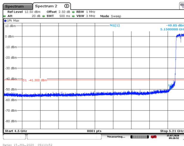
5230MHz with 4*4 CDD AV
