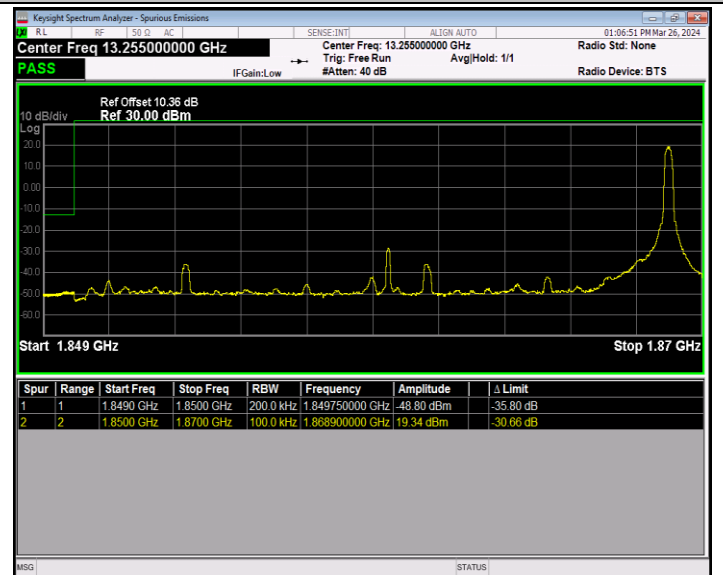
Band2_20MHz_QPSK_18700_1RB#99
