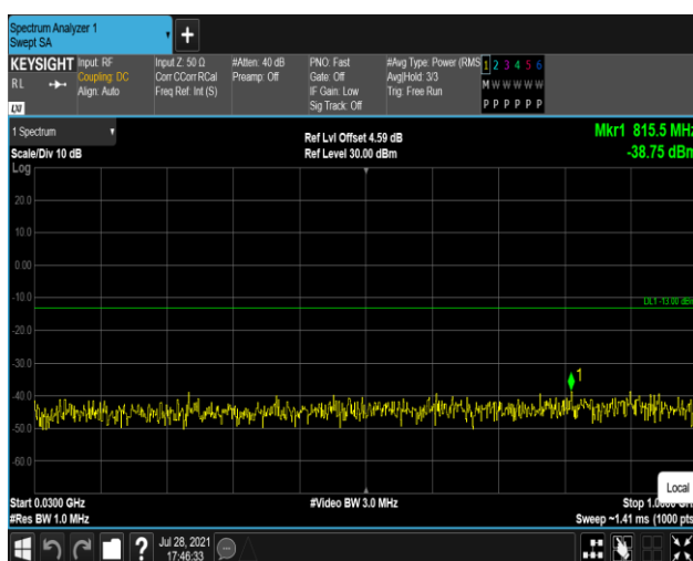
Band66-20MHz-QPSK-132322:30~1000MHz
