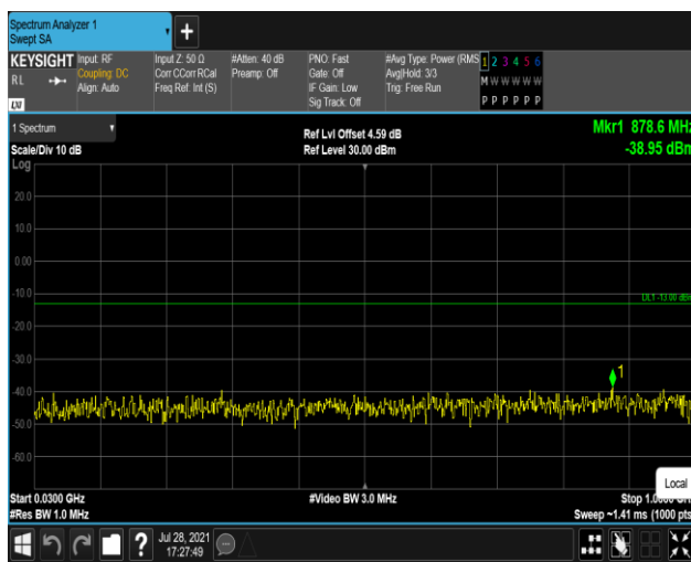
Band66-20MHz-QPSK-132072:30~1000MHz
