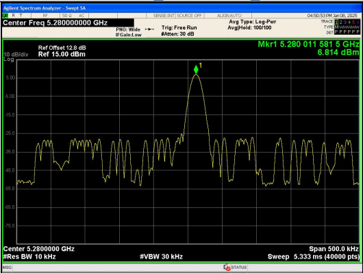
NT/NV_Antenna 0 IEEE 802.11n_Channel 56_20MHz
