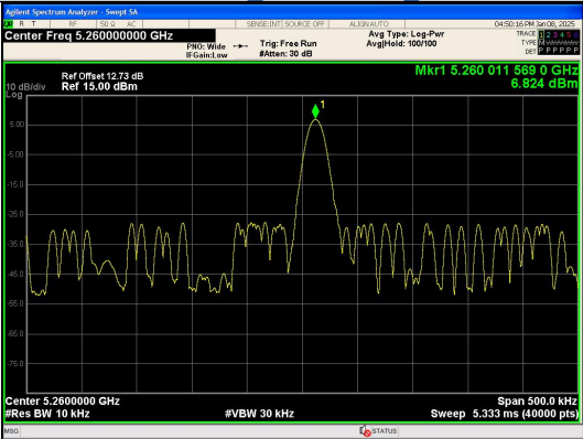
NT/NV_Antenna 0 IEEE 802.11n_Channel 52_20MHz
