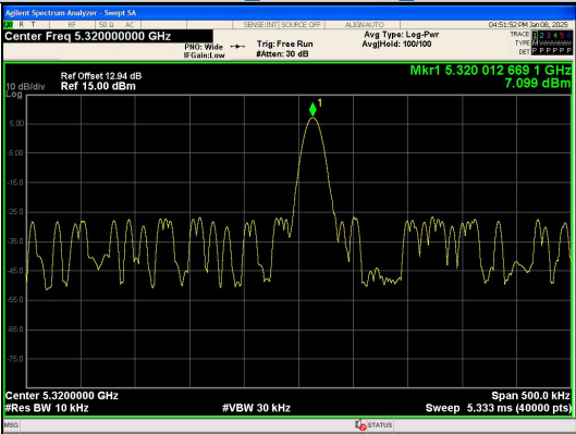
NT/NV_Antenna 0 IEEE 802.11n_Channel 64_20MHz
