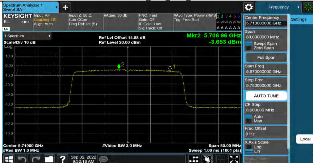
11AX40MIMO_Ant1 5710 UNII-3
