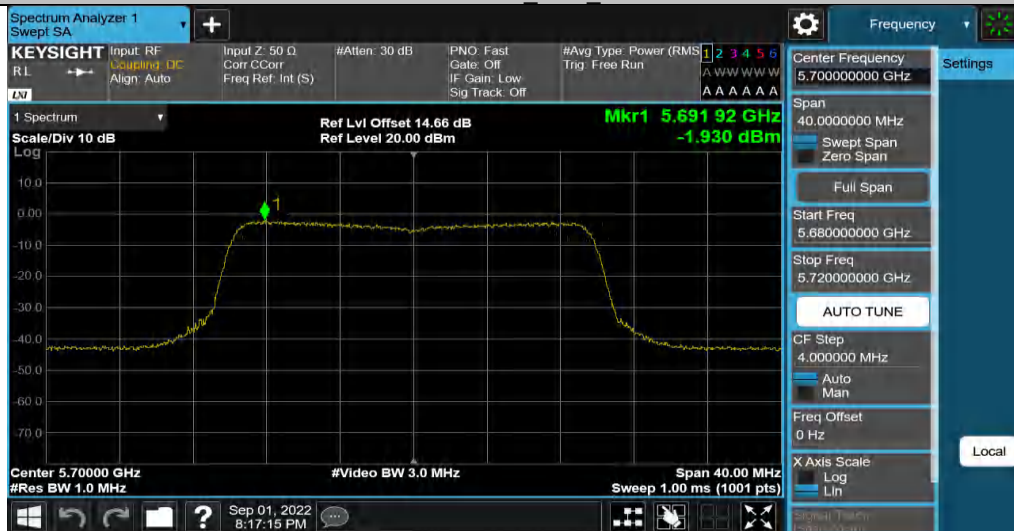
11AX20MIMO_Ant4_5700
