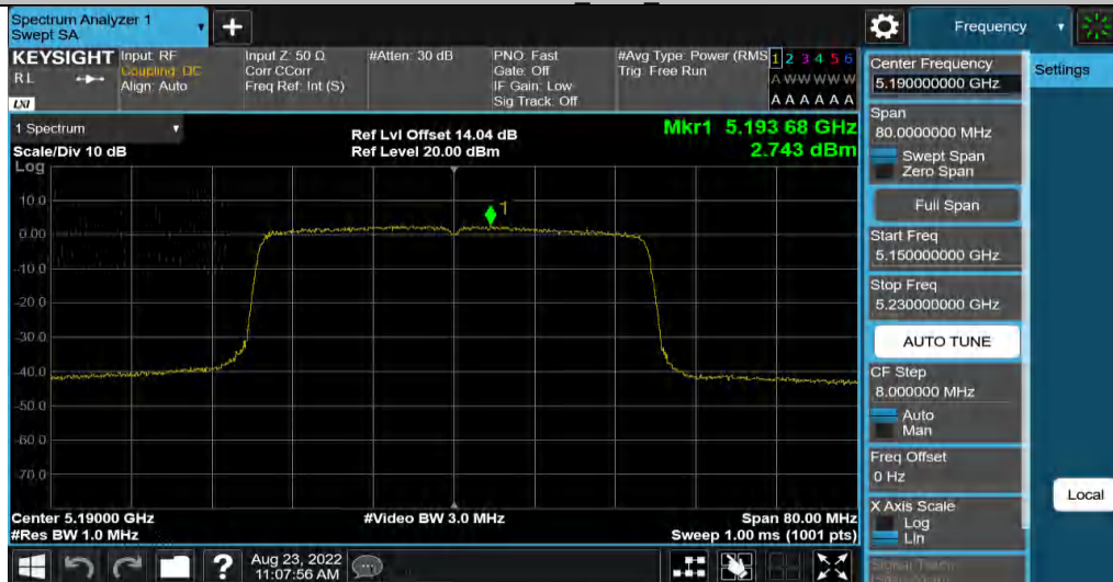
11AX40MIMO_Ant4_5190
