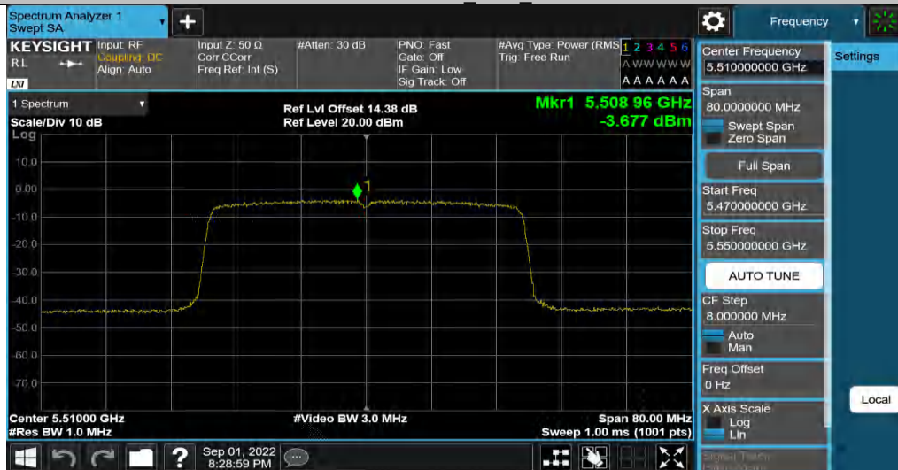
11AX40MIMO_Ant3_5510
