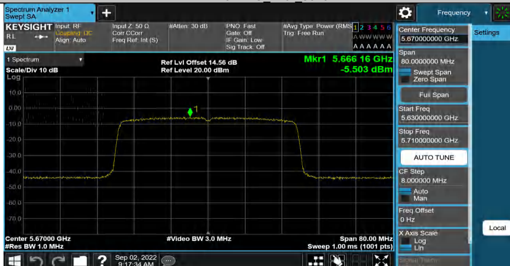
11AX40MIMO_Ant3_5670
