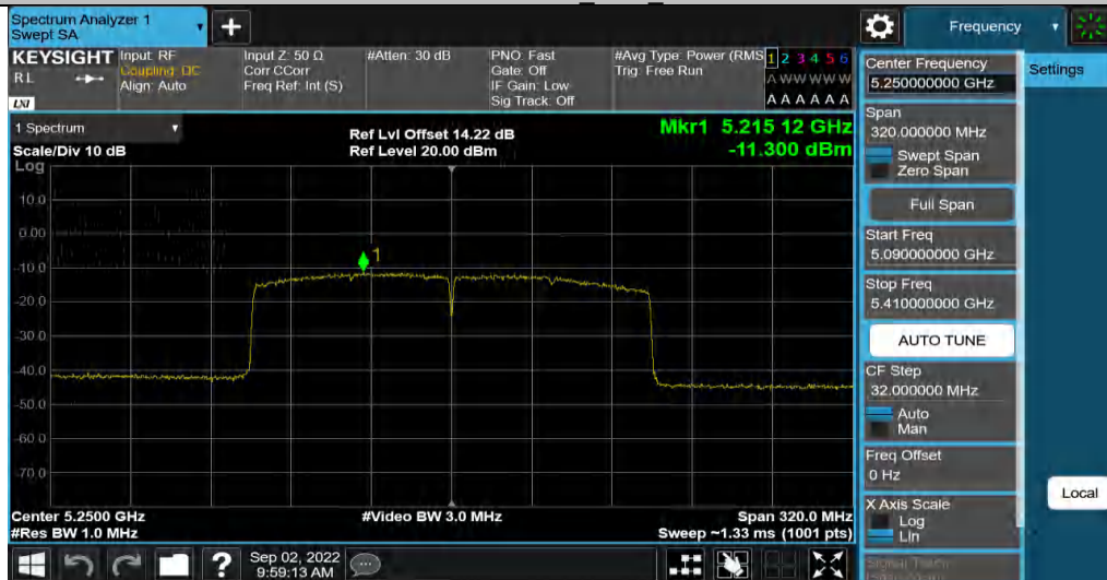
11AX160MIMO Ant4 5250
