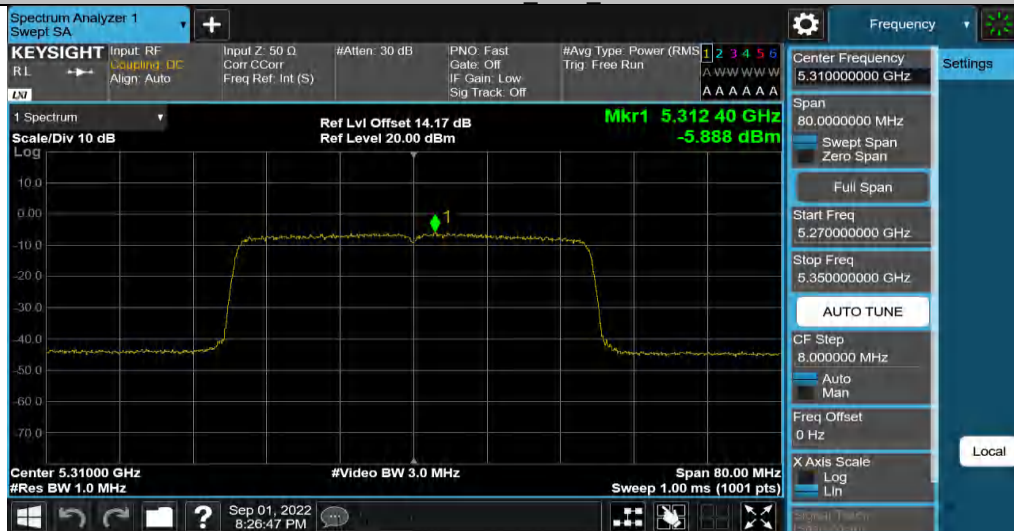
11AX40MIMO_Ant4_5310
