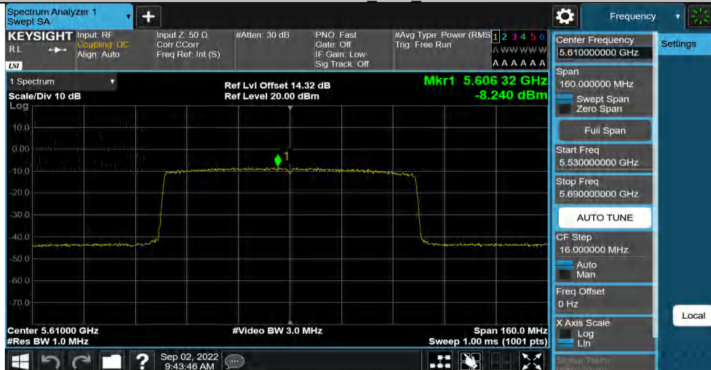
11AX80MIMO_Ant4_5610
