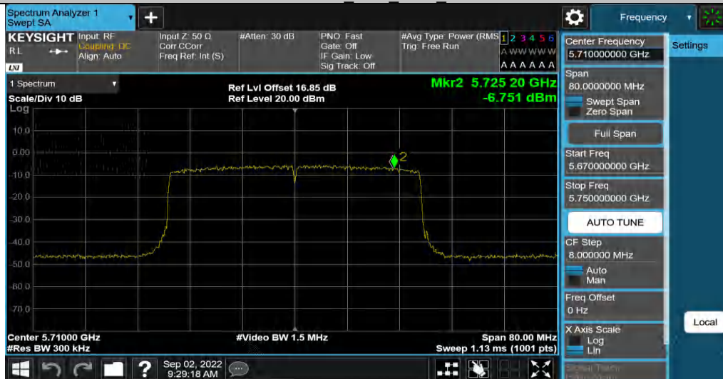
11AX40MIMO_Ant2 5710 UNII-3
