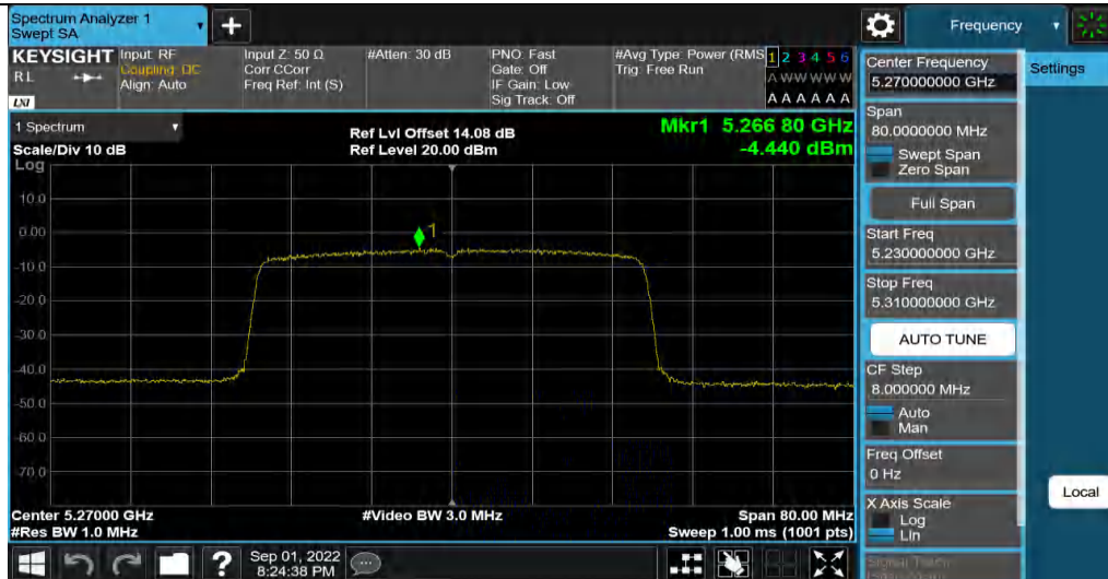
11AX40MIMO_Ant3_5270
