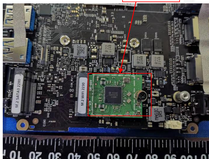
RF Module
