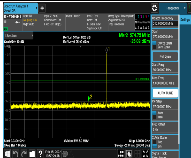
Band12-5MHz-QPSK-23035-1-0-Low-30-1000--35.08-PASS
