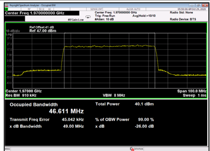
Figure 728: 256QAM 50MHz B.W.; 1970.0MHz, 60kHz - Output
