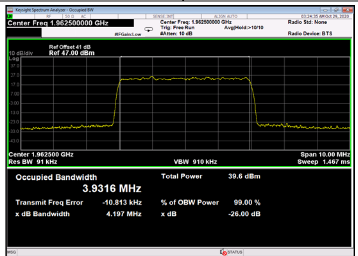
Figure 672: 256QAM 5MHz B.W.; 1962.5MHz, 30kHz - Output
