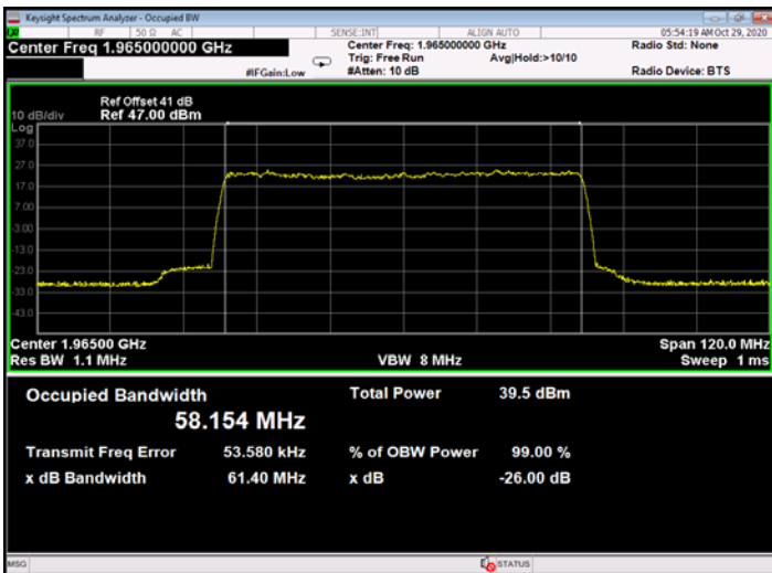
Figure 733: 256QAM 60MHz B.W.; 1965.0MHz, 30kHz - Output
