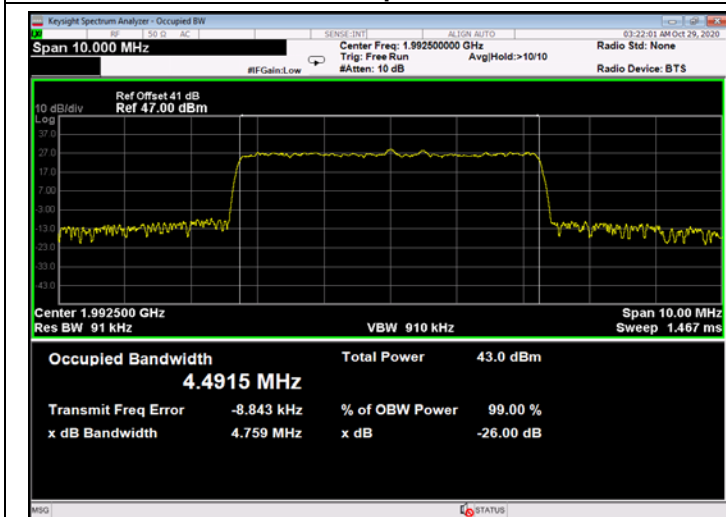
Figure 673: 256QAM 5MHz B.W.; 1992.5MHz, 15kHz - Output
