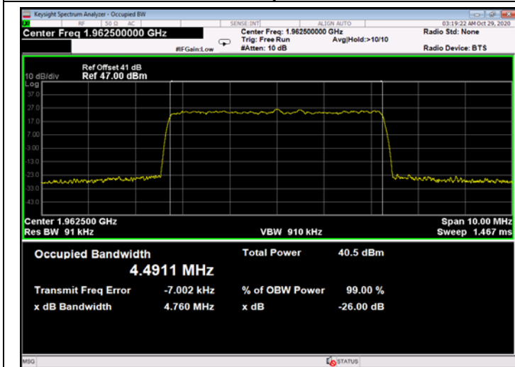
Figure 671: 256QAM 5MHz B.W.; 1962.5MHz, 15kHz - Output
