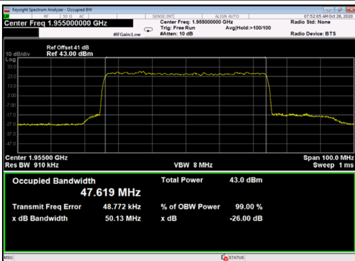
Figure 655: 64QAM 50MHz B.W.; 1955.0MHz, 30kHz - Output
