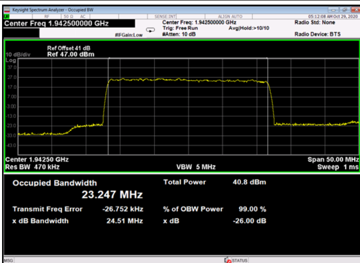
Figure 703: 256QAM 25MHz B.W.; 1942.5MHz, 30kHz - Output
