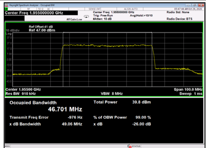
Figure 722: 64QAM 50MHz B.W.; 1955.0MHz, 60kHz - Output
