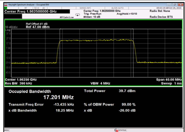
Figure 698: 256QAM 20MHz B.W.; 1962.5MHz, 60kHz - Output
