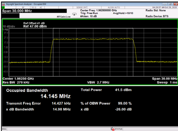
Figure 687: 256QAM 15MHz B.W.; 1962.5MHz, 15kHz - Output
