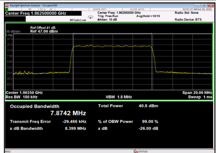
Figure 680: 256QAM 10MHz B.W.; 1962.5MHz, 60kHz - Output
