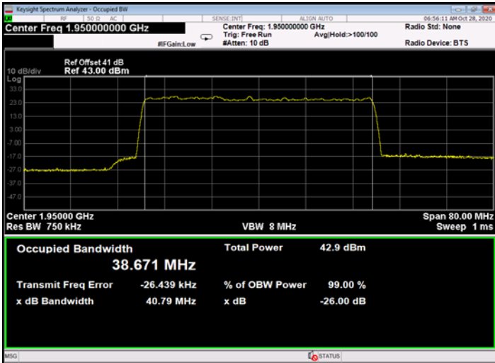
Figure 645: 64QAM 40MHz B.W.; 1950.0MHz, 15kHz - Output
