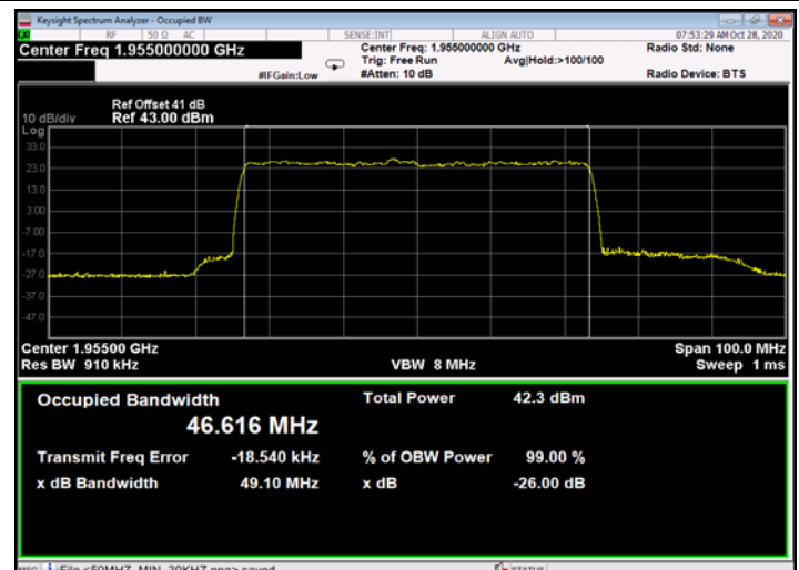
Figure 656: 64QAM 50MHz B.W.; 1955.0MHz, 60kHz - Output
