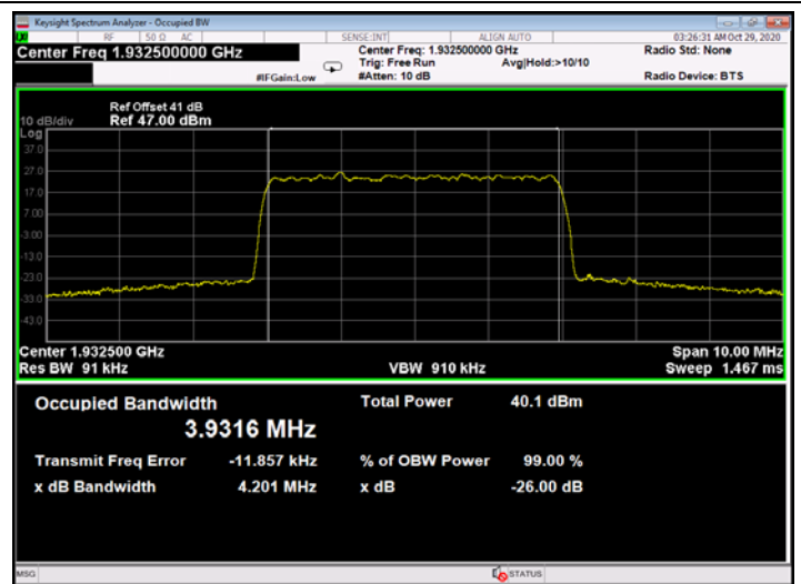
Figure 670: 256QAM 5MHz B.W.; 1932.5MHz, 30kHz - Output
