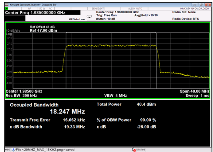
Figure 700: 256QAM 20MHz B.W.; 1985.0MHz, 30kHz - Output
