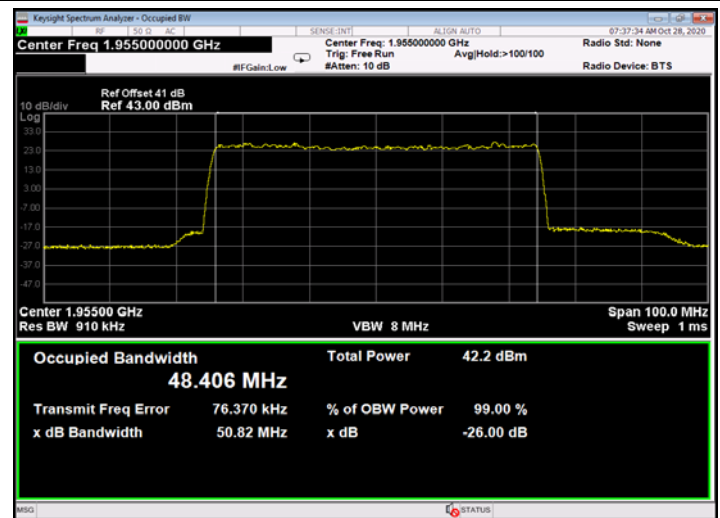
Figure 654: 64QAM 50MHz B.W.; 1955.0MHz, 15kHz - Output
