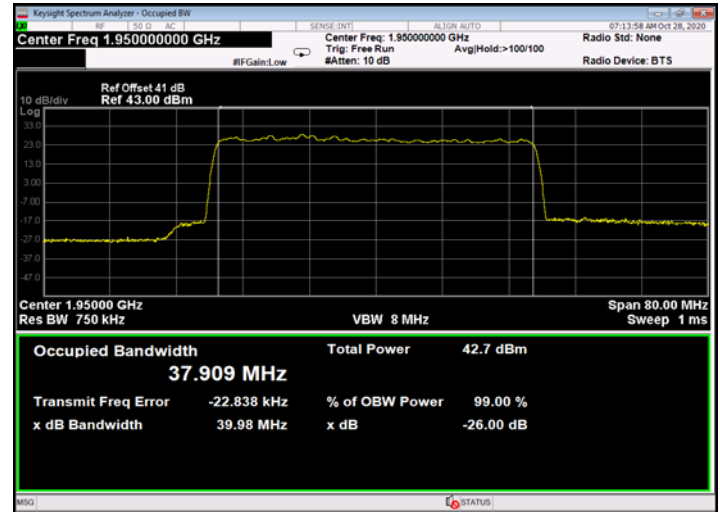
Figure 646: 64QAM 40MHz B.W.; 1950.0MHz, 30kHz - Output
