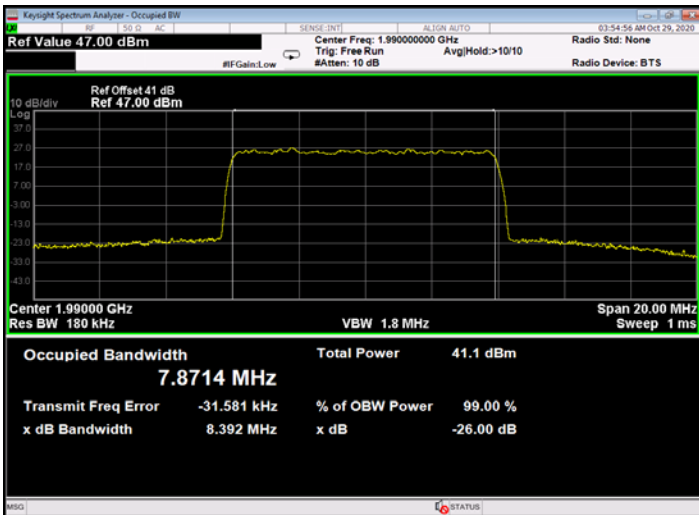
Figure 683: 256QAM 10MHz B.W.; 1990.0MHz, 60kHz - Output
