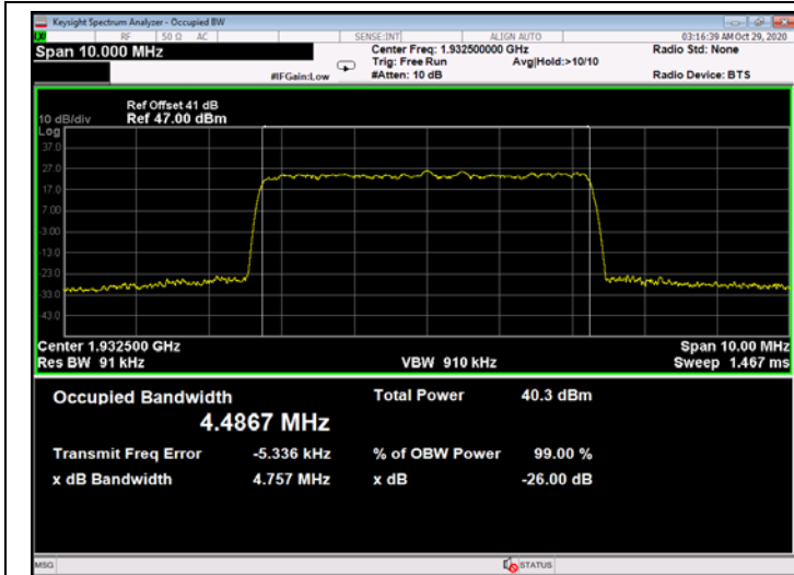
Figure 669: 256QAM 5MHz B.W.; 1932.5MHz, 15kHz - Output
