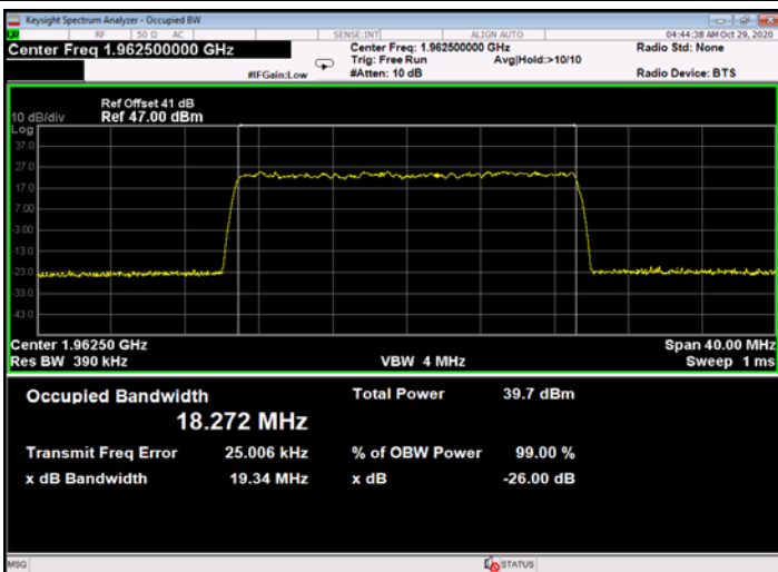
Figure 697: 256QAM 20MHz B.W.; 1962.5MHz, 30kHz - Output
