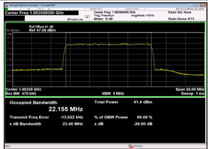
Figure 710: 256QAM 25MHz B.W.; 1982.5MHz, 60kHz - Output
