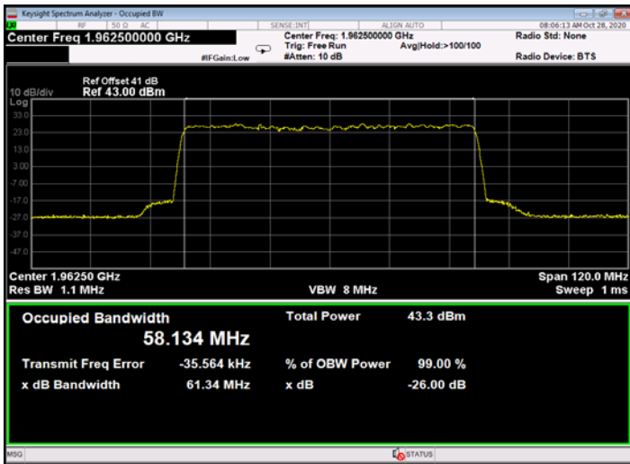
Figure 665: 64QAM 60MHz B.W.; 1962.5MHz, 30kHz - Output
