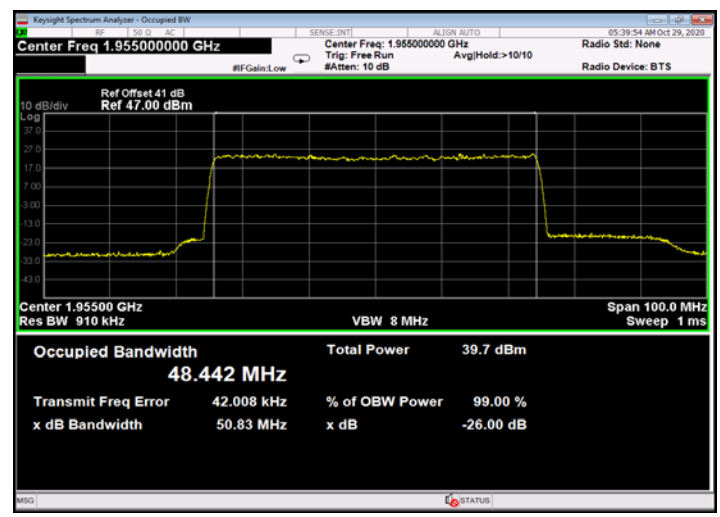
Figure 720: 256QAM 50MHz B.W.; 1955.0MHz, 15kHz - Output
