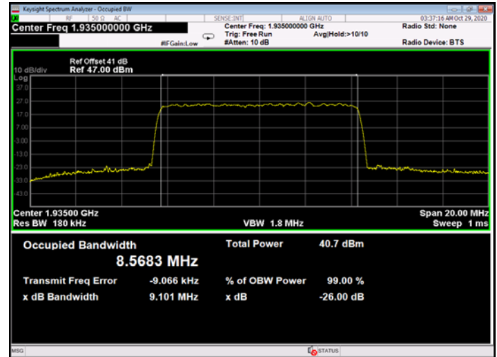
Figure 676: 256QAM 10MHz B.W.; 1935.0MHz, 30kHz - Output
