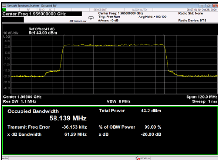
Figure 667: 64QAM 60MHz B.W.; 1965.0MHz, 30kHz - Output
