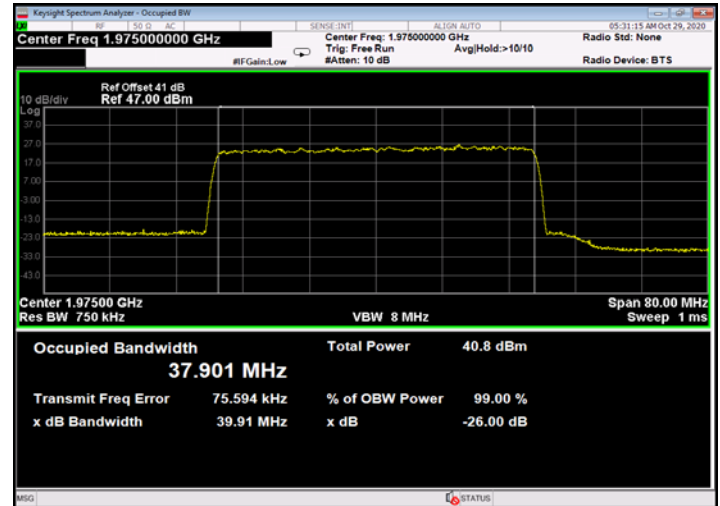
Figure 718: 256QAM 40MHz B.W.; 1975.0MHz, 30kHz - Output
