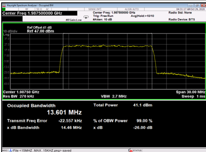
Figure 691: 256QAM 15MHz B.W.; 1987.5MHz, 30kHz - Output
