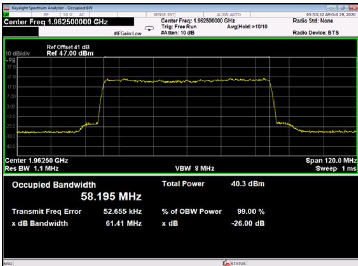
Figure 731: 256QAM 60MHz B.W.; 1962.5MHz, 30kHz - Output
