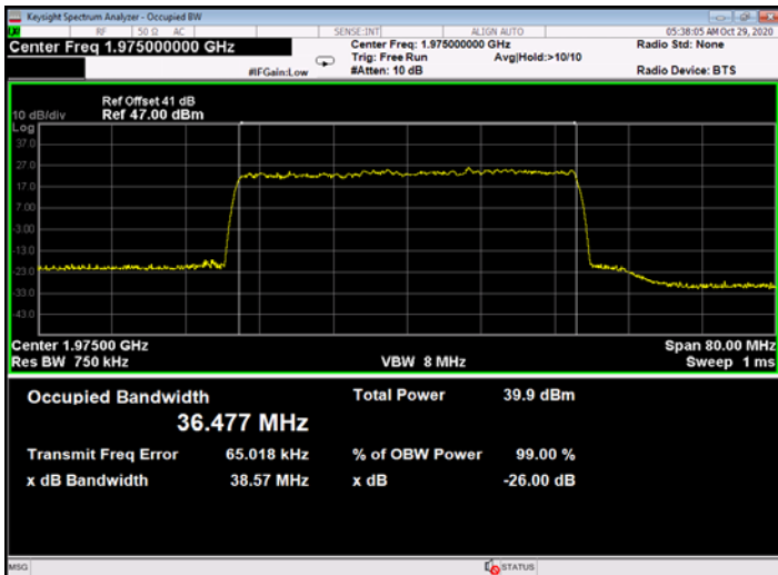
Figure 719: 256QAM 40MHz B.W.; 1975.0MHz, 60kHz - Output
