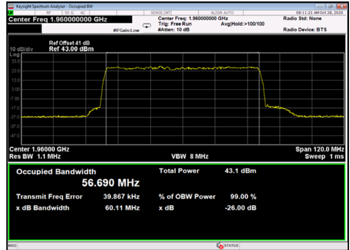
Figure 664: 64QAM 60MHz B.W.; 1960.0MHz, 60kHz - Output
