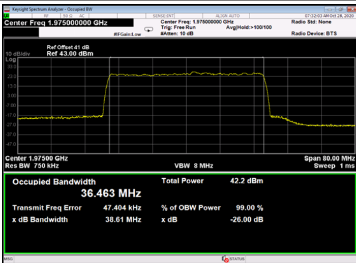
Figure 653: 64QAM 40MHz B.W.; 1975.0MHz, 60kHz - Output
