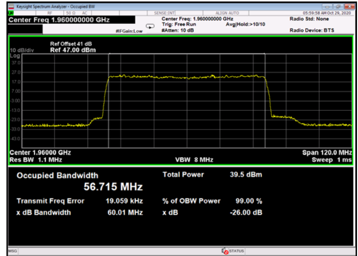
Figure 730: 256QAM 60MHz B.W.; 1960.0MHz, 60kHz - Output
