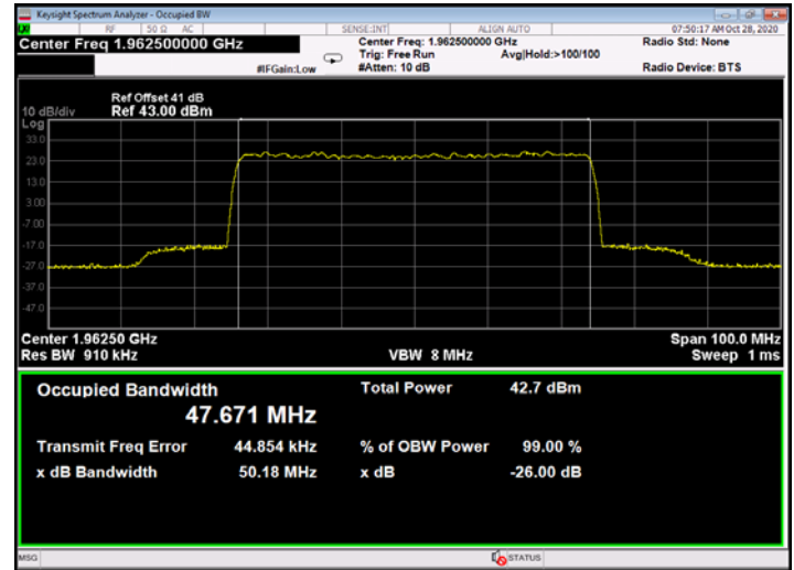
Figure 658: 64QAM 50MHz B.W.; 1962.5MHz, 30kHz - Output
