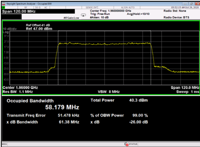
Figure 729: 256QAM 60MHz B.W.; 1960.0MHz, 30kHz - Output
