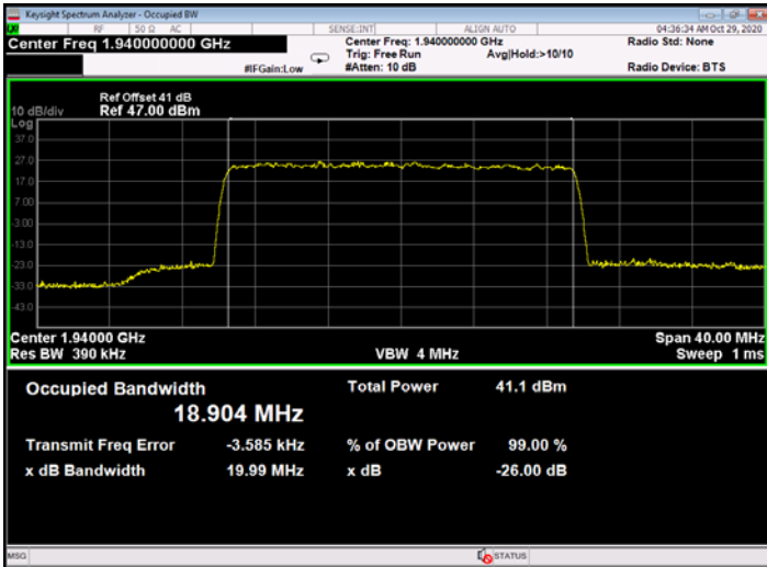
Figure 693: 256QAM 20MHz B.W.; 1940.0MHz, 15kHz - Output
