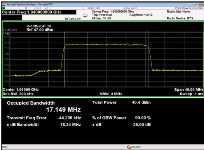
Figure 695: 256QAM 20MHz B.W.; 1940.0MHz, 60kHz - Output
