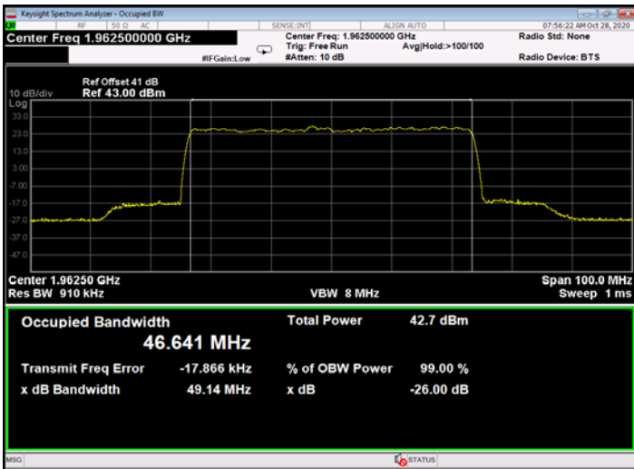
Figure 659: 64QAM 50MHz B.W.; 1962.5MHz, 60kHz - Output
