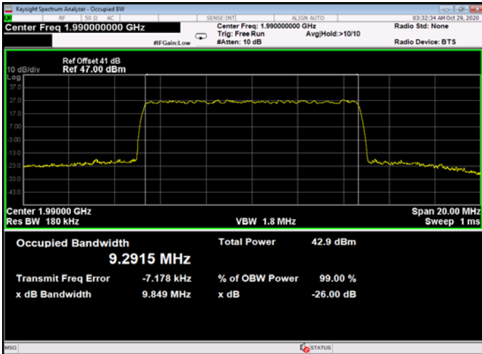
Figure 681: 256QAM 10MHz B.W.; 1990.0MHz, 15kHz - Output
