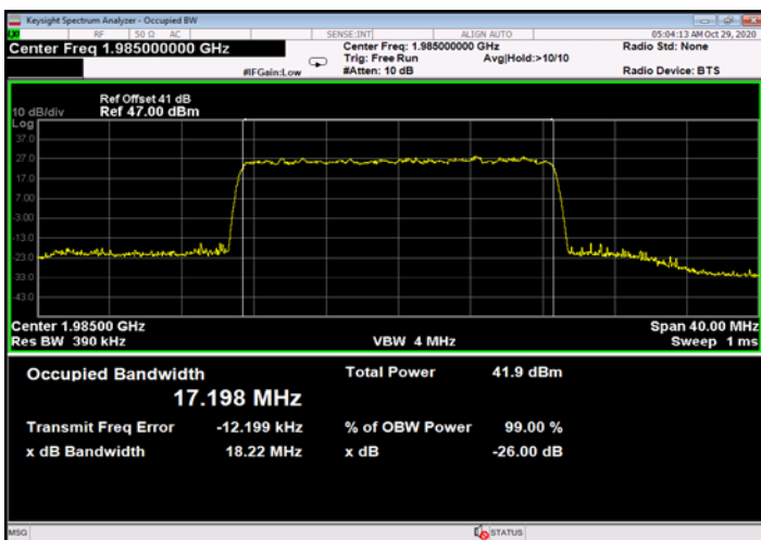
Figure 701: 256QAM 20MHz B.W.; 1985.0MHz, 60kHz - Output
