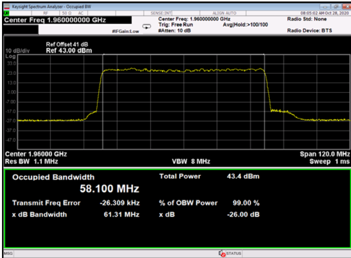
Figure 663: 64QAM 60MHz B.W.; 1960.0MHz, 30kHz - Output
