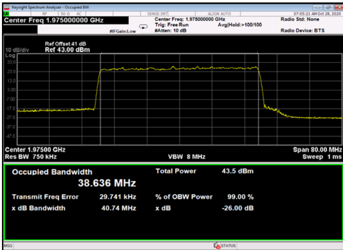
Figure 651: 64QAM 40MHz B.W.; 1975.0MHz, 15kHz - Output
