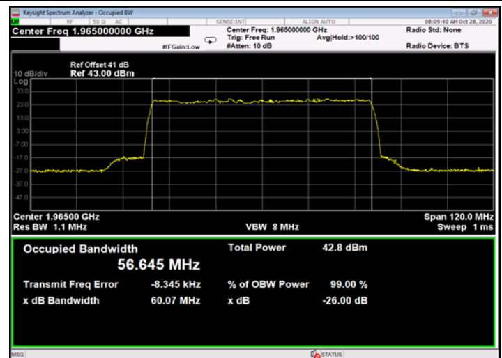
Figure 668: 64QAM 60MHz B.W.; 1965.0MHz, 60kHz - Output
