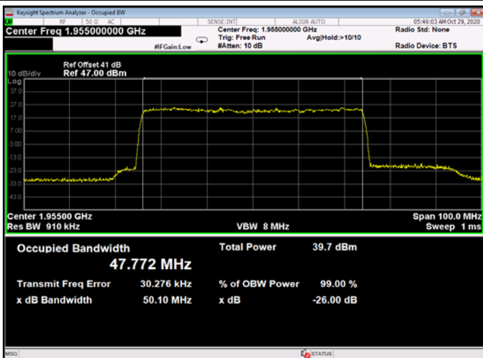
Figure 721: 256QAM 50MHz B.W.; 1955.0MHz, 30kHz - Output
