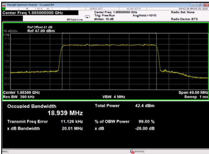
Figure 699: 256QAM 20MHz B.W.; 1985.0MHz, 15kHz - Output
