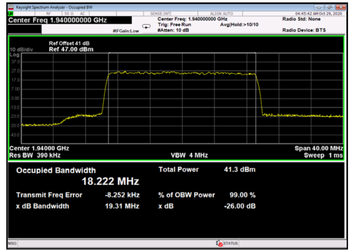
Figure 694: 256QAM 20MHz B.W.; 1940.0MHz, 30kHz - Output
