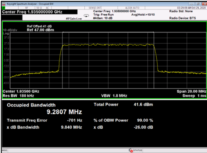
Figure 675: 256QAM 10MHz B.W.; 1935.00MHz, 15kHz - Output
