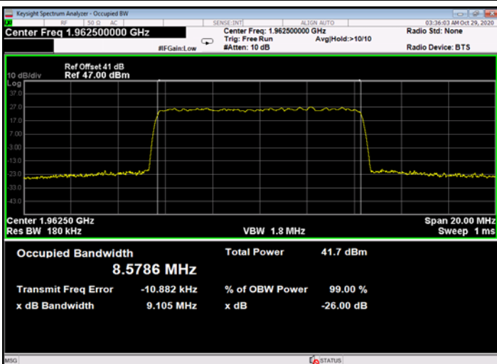
Figure 679: 256QAM 10MHz B.W.; 1962.5MHz, 30kHz - Output
