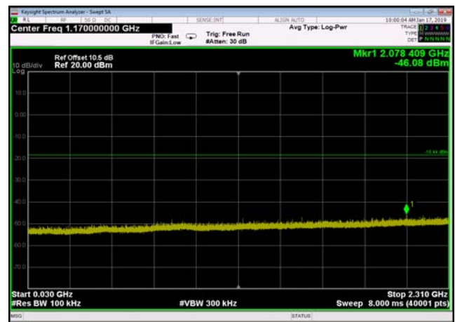
,Plot 3,30MHz~2310MHz-802.11g,2462MHz ,Ant0
