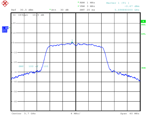
802.11n20_5700MHz
