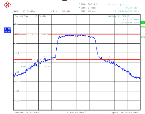
802.11n20_5720MHz 29.949MHz
