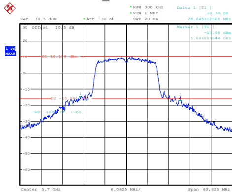
802.11n20_5700MHz 28.645MHz
