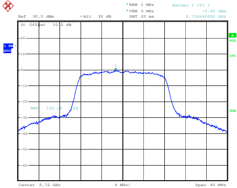
802.11a_5720MHz
