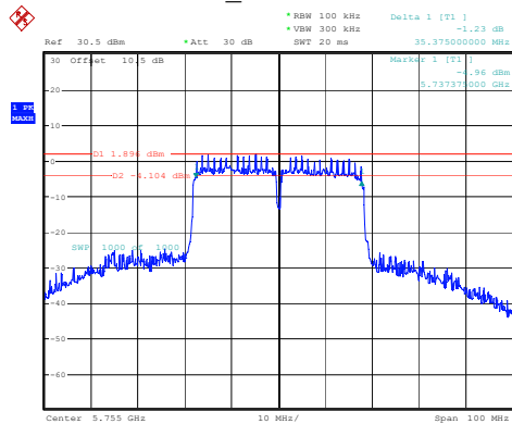
802.11n40_5755MHz 35.375MHz
