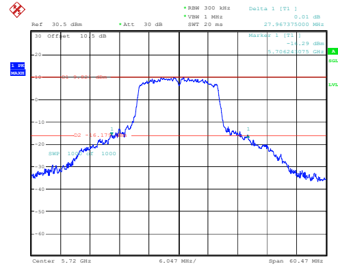
802.11a_5720MHz 27.967MHz
