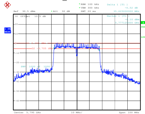
802.11n40_5795MHz 35.625MHz
