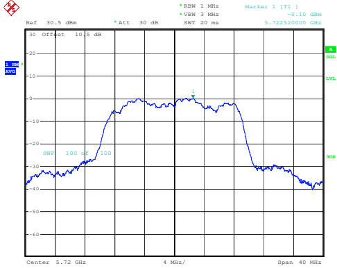
802.11n20_5720MHz
