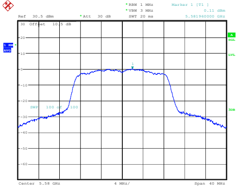
802.11n20_5580MHz
