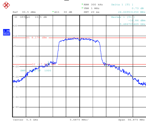
802.11n20_5500MHz 24.670MHz
