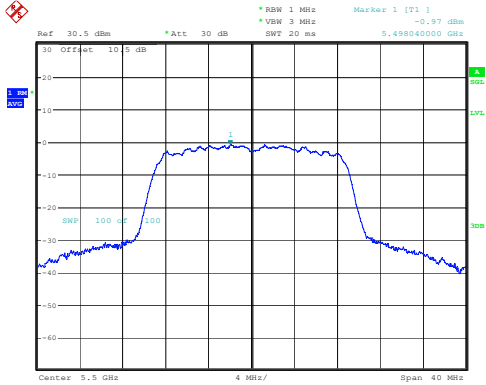
802.11n20_5500MHz
