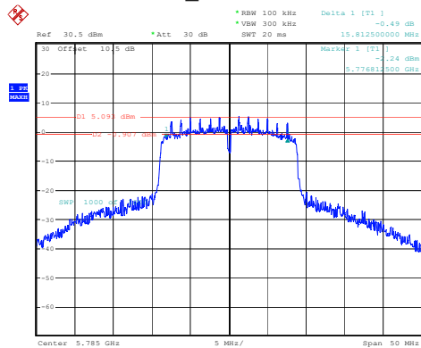
802.11n20_5785MHz 15.813MHz
